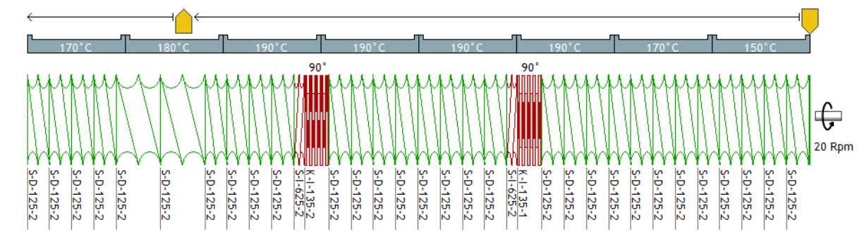
Figure III.32: Profil de vis d'extrusion et de température
