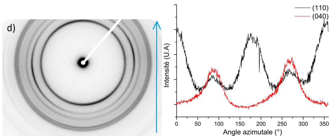
Figure A.52 : Cliché WAXS 2D du CA 100 T3000 1:1 déformé à \varepsilon_{33}=0,9 et profile azimutale des plans de diffraction (110) et (040) du polypropylène.
