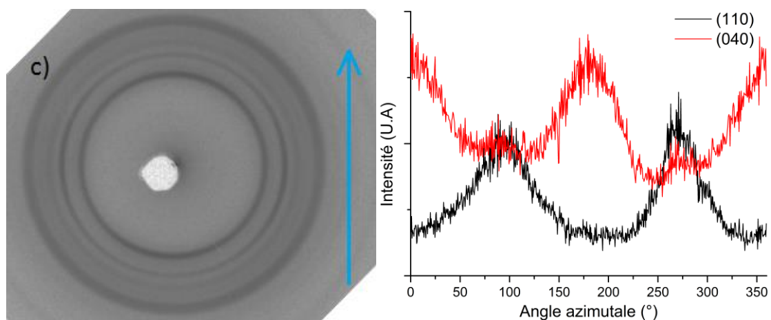
Figure A.43: Cliché WAXS 2D du CA 100 THF 100 1 :1 KNG 180 traité 5% m et profile azimutale des plans de diffraction (110) et (040) du polypropylène.
