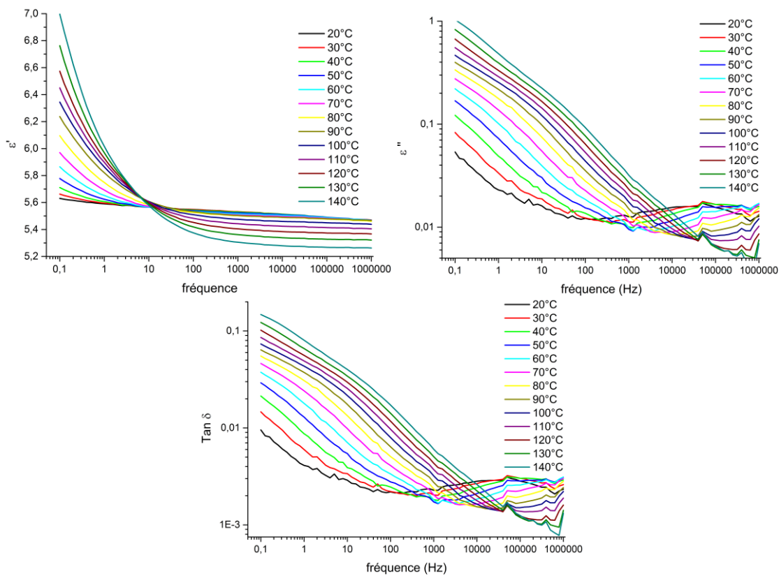
Figure A.61 : Spectre diélectrique \epsilon' , \epsilon'' , et Tan \delta en fonction de la fréquence du matériau CA 100 THF 100 1:1 KNG 180 1% m
