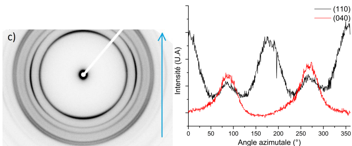
Figure A.51 : Cliché WAXS 2D du CA 100 T3000 1:1 déformé à \varepsilon_{33}=0,6 et profile azimutale des plans de diffraction (110) et (040) du polypropylène.
