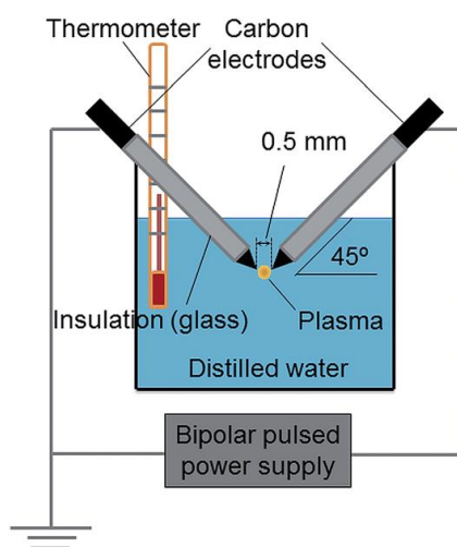
Figure 1.28: Montage expérimental pour l'exfoliation du graphène à partir d'électrodes de graphite par Lee et al. , 2014 [280].
