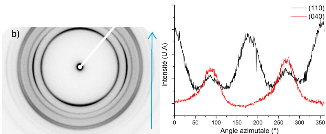
Figure A.50 : Cliché WAXS 2D du CA 100 T3000 1:1 déformé à \varepsilon_{33}=0,3 et profile azimutale des plans de diffraction (110) et (040) du polypropylène.
