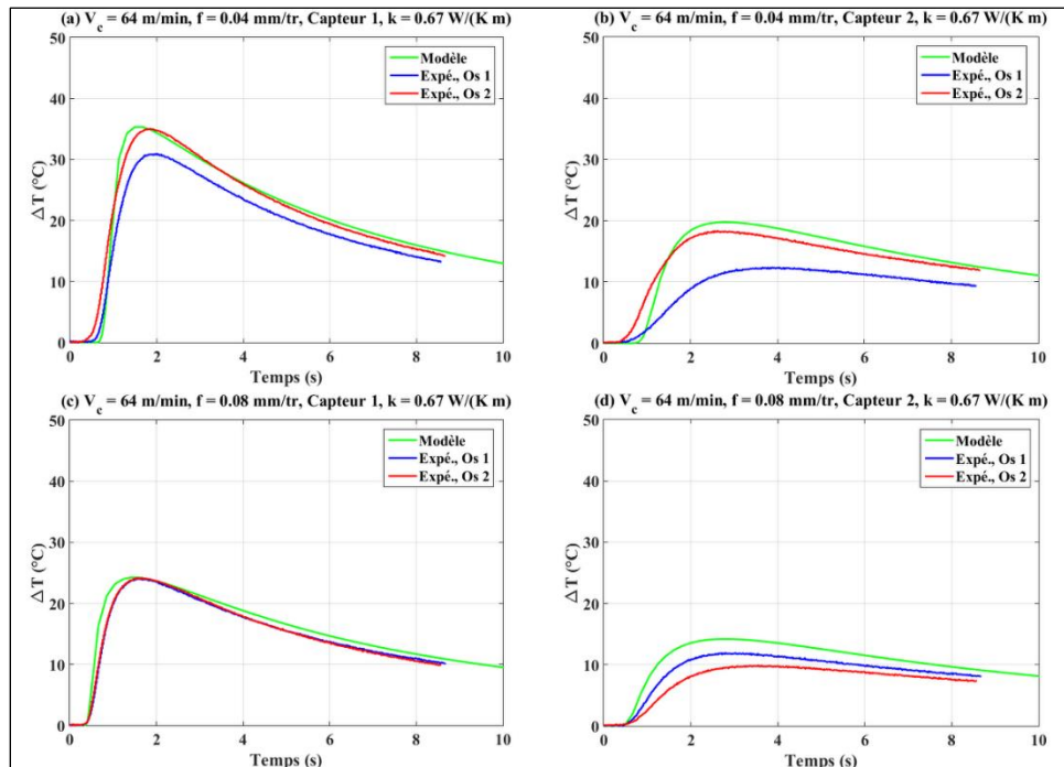
Figure 4-17 : Comparaison résultats du modèle analytique ( k = 0.67 \text{ W/(K m)} ) vs résultats expérimentaux ( V_c = 64 \text{ m/min} , d = 4 \text{ mm} )
