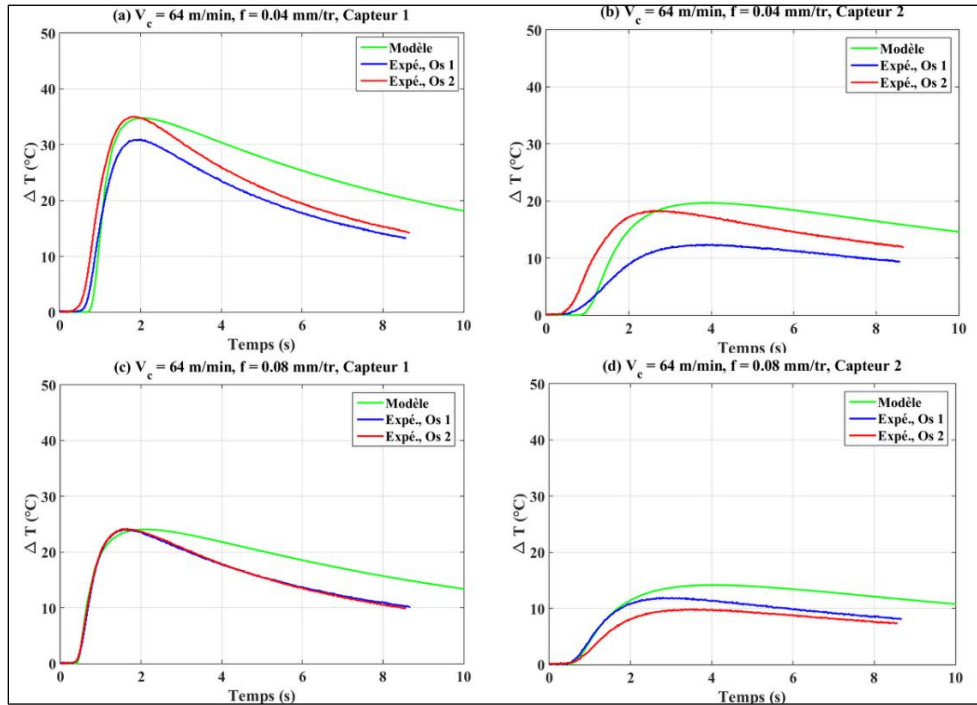
Figure 4-15 : Comparaison résultats du modèle analytique vs résultats expérimentaux ( V_c = 64 \text{ m/min} , d = 4 \text{ mm} )
