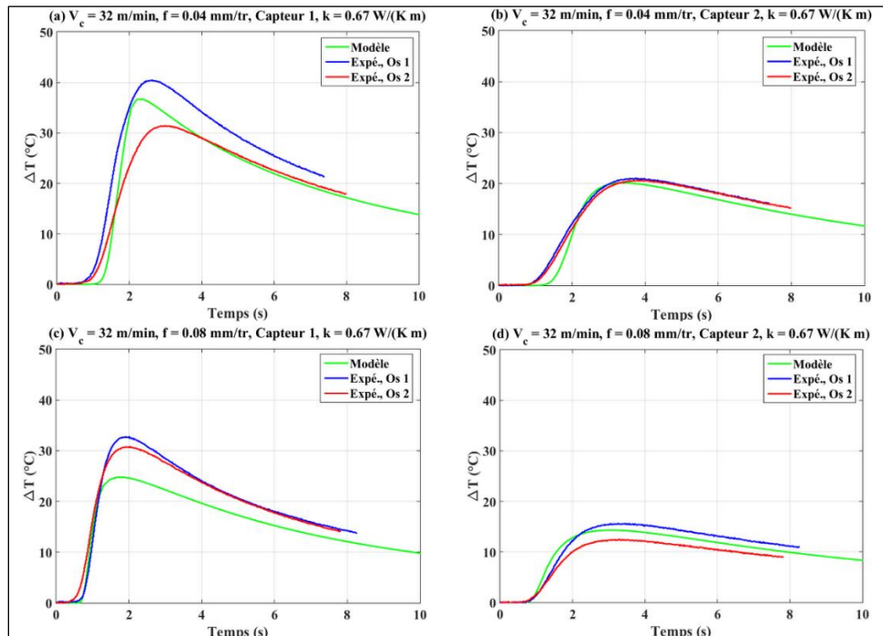
Figure 4-16 : Comparaison résultats du modèle analytique ( k = 0.67 \text{ W/(K m)} ) vs résultats expérimentaux ( V_c = 32 \text{ m/min} , d = 4 \text{ mm} )
