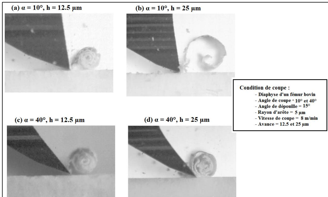
Figure 3-7 : Morphologie de copeaux suivant l'angle de coupe de l'outil et la profondeur de coupe (Feldmann et al., 2017)
