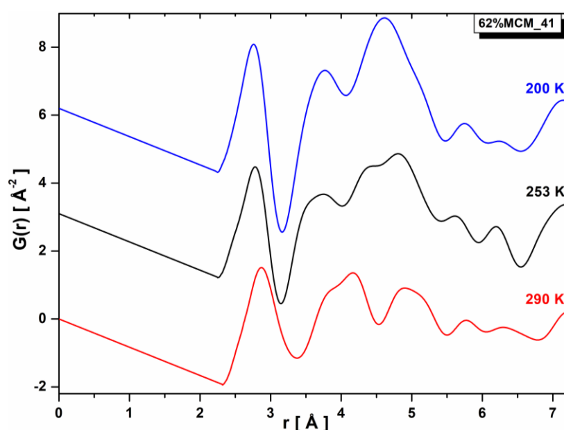
Figure V-23: Fonctions de distribution de paires différentielles, d-PDF, G(r) de l'eau confinée dans le MCM-41 avec un taux de 62%, en fonction de la température.
