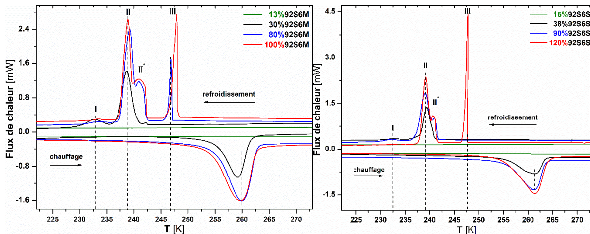
Figure IV-9: Mesures DSC pour l'eau confinée avec différents taux de remplissage des pores dans: le 92S6M (A gauche) et le 92S6S (A droite).
