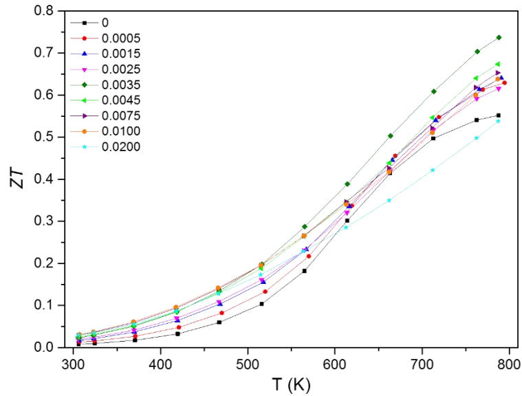
Figure 2 : Dépendance en température du facteur de mérite thermoélectrique adimensionnel ZT pour les échantillons \text{Sn}_{1.03-x}\text{In}_x\text{Te} ( 0.0 \leq x \leq 0.02 ).
