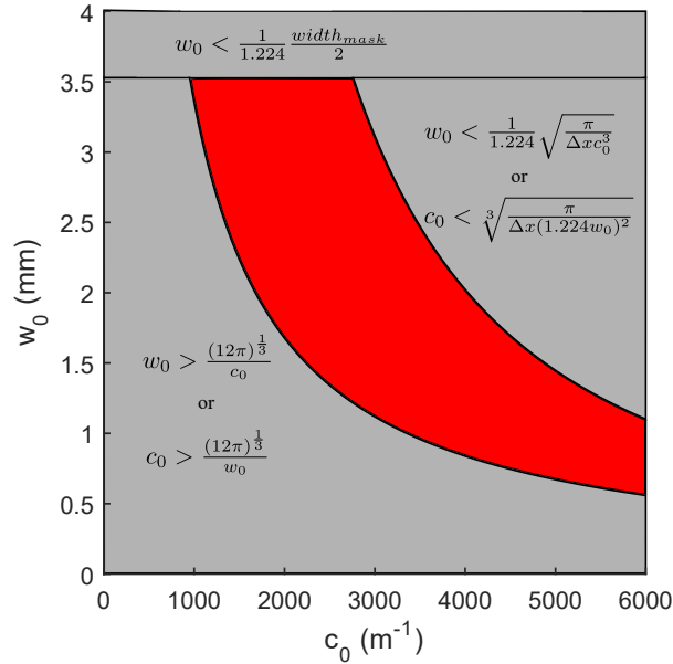
Figure 6.6: Graphique représentant en rouge la plage de paramètres permettant la génération de faisceaux Airy. w_0 est la taille du faisceau Gaussien éclairant le masque de phase et c_0 représente le déphasage maximal au sein du masque.
