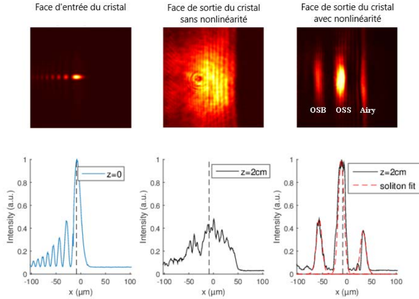
Figure 6.7: De gauche à droite : face d'entrée du cristal où l'on injecte un faisceau Airy unidimensionnel, face de sortie du cristal sans nonlinéarité présentant un faisceau Airy diffus, face de sortie du cristal avec nonlinéarité présentant un OSB, OSS et faisceau Airy résiduel.
