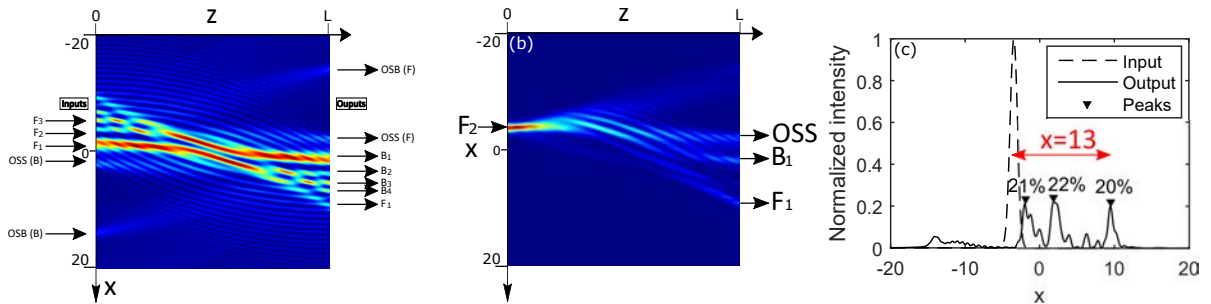
Figure 6.10: (a) Profil d'intensité à l'intérieur du cristal représentant la structure du guide d'onde créée par deux faisceaux Airy contrapropageant antisymétriquement. Les flèches de gauche représentent des entrées et les flèches de droite des sorties. (b) Propagation d'un faisceau Gaussien dans le guide d'onde injecté dans l'entrée F_2 . (c) Profil d'intensité transverse à la sortie du guide d'onde pour un faisceau Gaussien injecté dans l'entrée F_2 , en rouge est représenté le décalage maximal entre la position du faisceau d'entrée et la sortie la plus décalée correspond à 13 tailles de faisceau.
