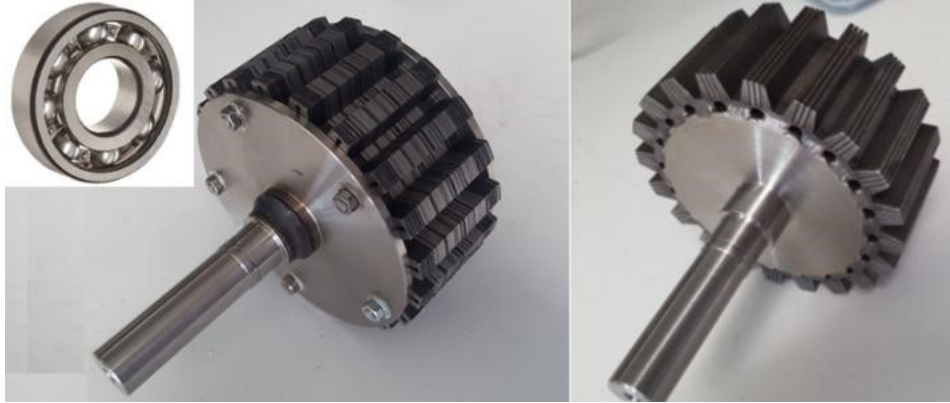
Figure IV.11. Deux versions du rotor et des roulements utilisés.
