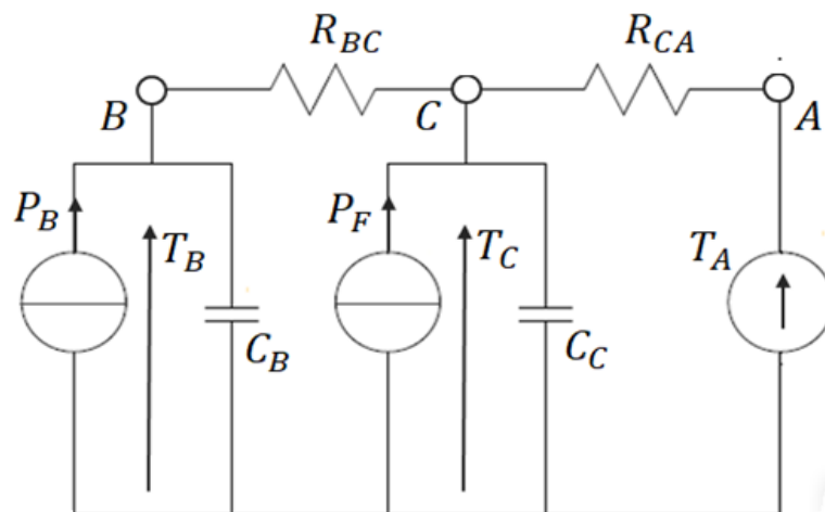
Figure IV.38. Schéma équivalent thermique complété pour prendre en compte les pertes dans les bobines et leur évacuation au travers du stator.
