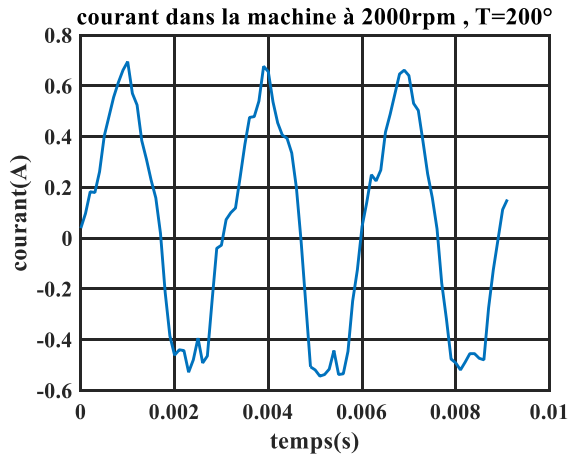
L'onde du courant 1 phase à 2000 rpm, T=200°C
