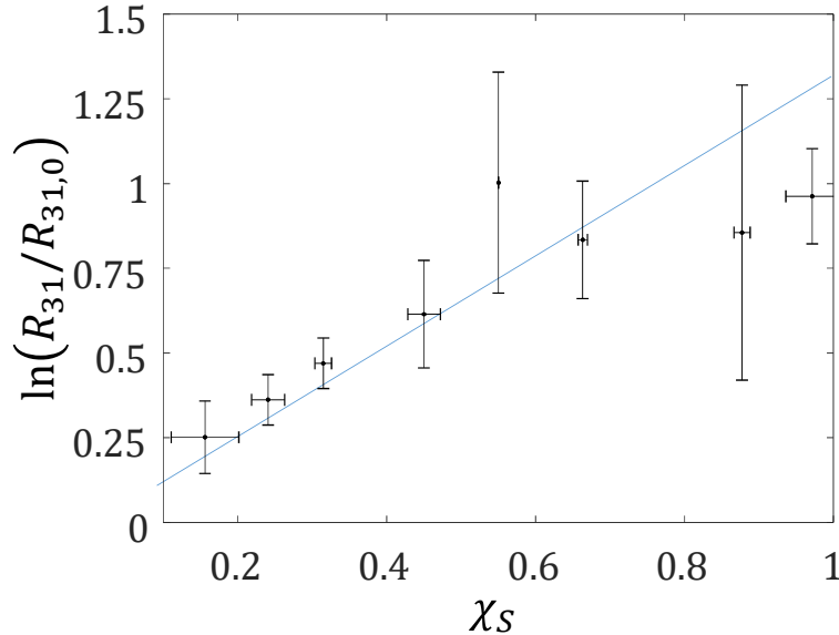
FIGURE 3.32 – Évolution du logarithme du rapport de fluorescence \ln(R_{31}/R_{31,0}) en fonction de la fraction de glace reconstruite grâce à la technique d'IRMN
