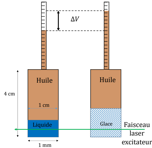
FIGURE 3.21 – cuvette jaugée utilisée pour la calibration du signal de fluorescence en fonction de la variation de volume d’eau, lors de la phase de solidification.
