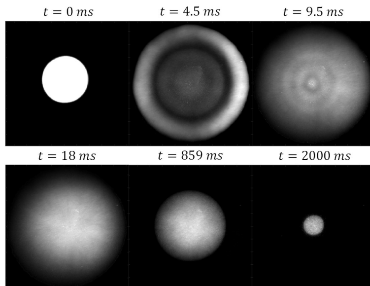
FIGURE 5.6 – Image de fluorescence d'une goutte impactant un substrat de Duraluminium sous-refroidi à -10\text{ }^{\circ}\text{C} à humidité non contrôlée. La température initiale de la goutte est de 18\text{ }^{\circ}\text{C} et le nombre de Weber d'impact est de 65. Les images ont été obtenues avec le dispositif de la Figure 5.2.
