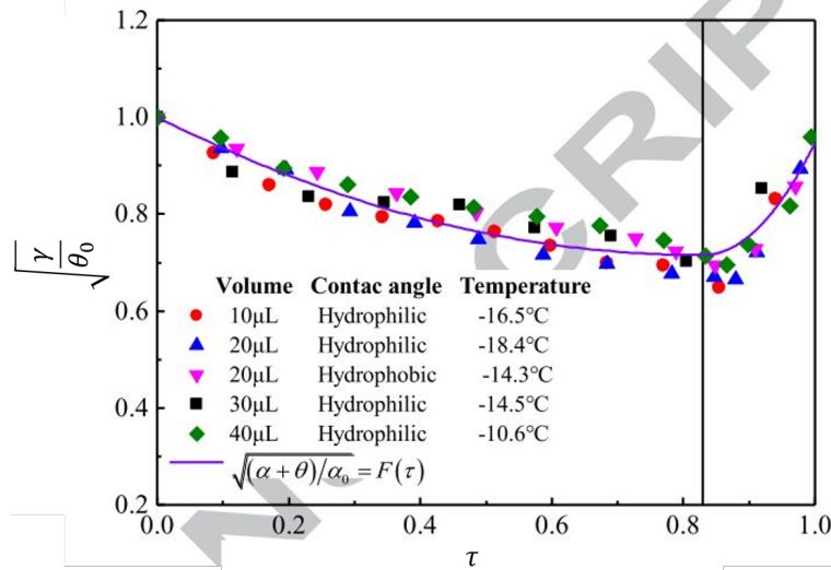
FIGURE 2.18 – Évolution de la racine carré l'angle de contact \gamma ( \gamma = \alpha + \theta ) en fonction du temps normalisé. L'ajustement des résultats expérimentaux par l'équation 2.54 est ajouté [74].
