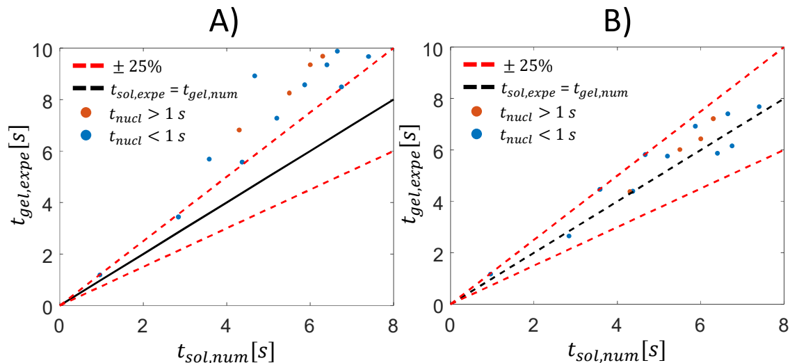
FIGURE 5.43 – Comparaisons entre les temps de solidifications obtenus expérimentalement et numériquement dans le cas A) de la modélisation 1D semi-infini (section 5.3.1.1) et dans le cas B) du modèle développé dans les sections 5.4.1.1 et 5.4.1.2.
