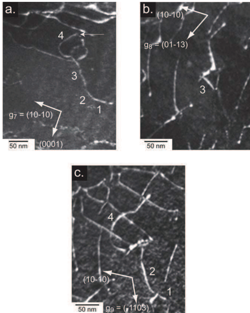
Figure V.13 – Micrographies MET de la configuration F ; a. avec g_7 = (10\bar{1}0) ; b. avec g_8 = (01\bar{1}3) et c. avec g_9 = (\bar{1}103) . La flèche localise l'interaction avec la partie 4.
