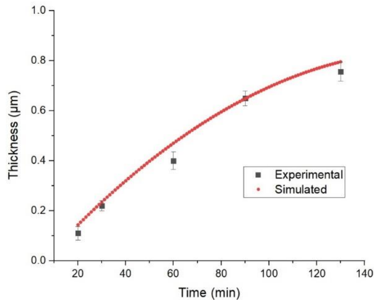
Fig. 4: Comparaison des mesures expérimentales de l'épaisseur de films de ZnO préparés par évaporation réactive en fonction du temps de dépôt, avec leurs valeurs simulées correspondantes. Les valeurs du point 0 m sur l'axe r et 0,0930 m sur l'axe z ont été utilisées pour calculer l'épaisseur.
