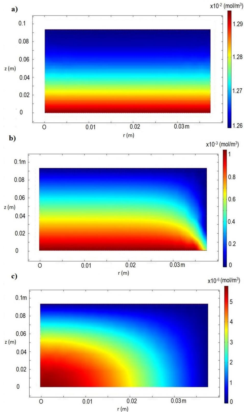
Fig. 2: Simulation du profil de distribution de la concentration de l'espèce a) O_2 , b) Zn , et c) ZnO . Dans l'axe r : 0 m est le centre du substrat et 0,0375 m est le bord du substrat; dans l'axe z : 0 m est le trou de la cellule Knudsen et 0,0930 m est la surface du substrat.
