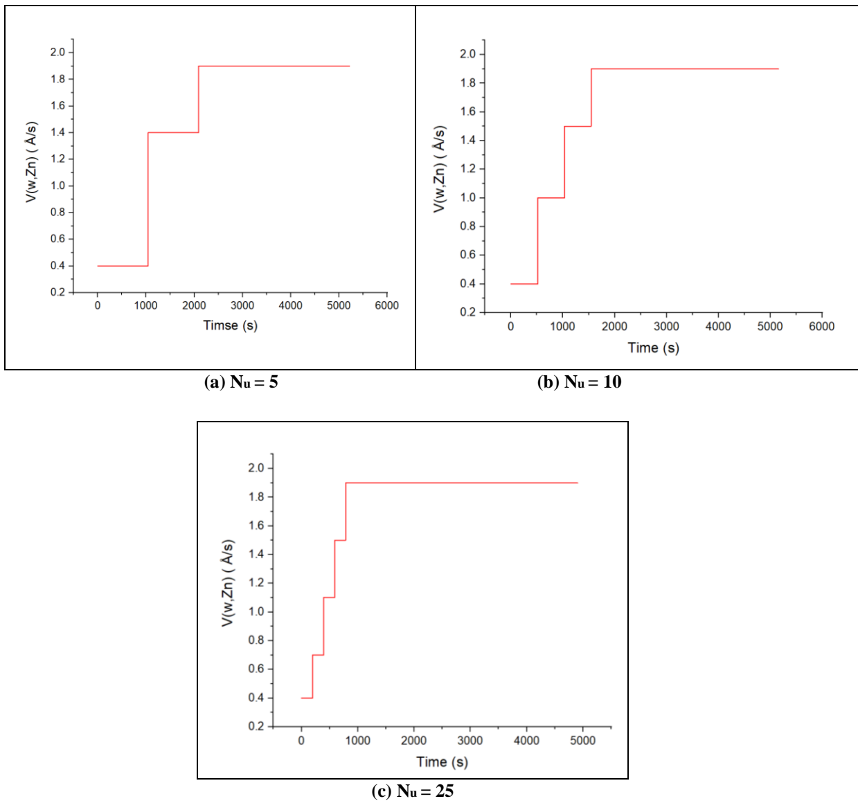
Figure 5.1 Profil d'écoulement optimal de Zn pour la minimisation du temps
