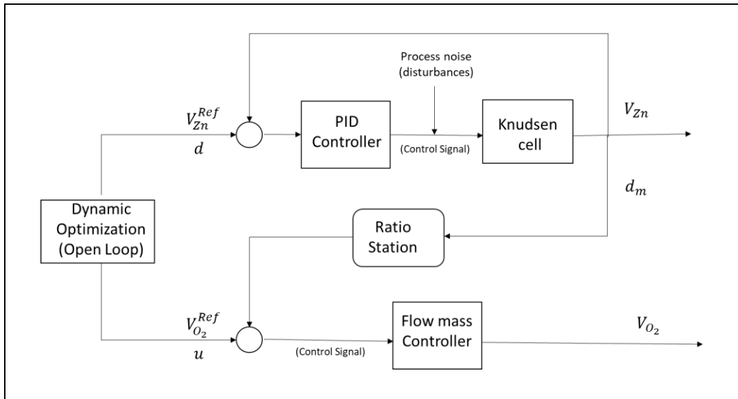
Figure 6.7: Représentation schématique du contrôle RC de simulation du processus d'évaporation réactive assistée par plasma.
