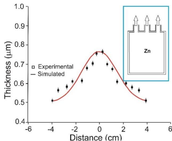
Fig. 3: Profil d'épaisseur de film final expérimental et simulé d'un film de ZnO typique. L'encart montre une cellule Knudsen avec une conception qui permettrait d'obtenir plus d'homogénéité dans l'épaisseur des films de ZnO.
