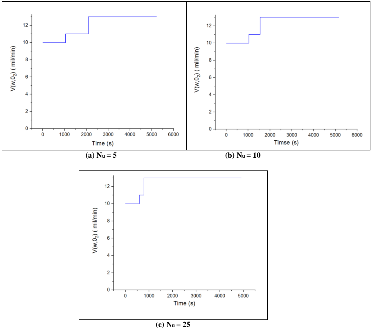
Figure 5.2 Profil de débit d'O 2 optimal pour la minimisation du temps
