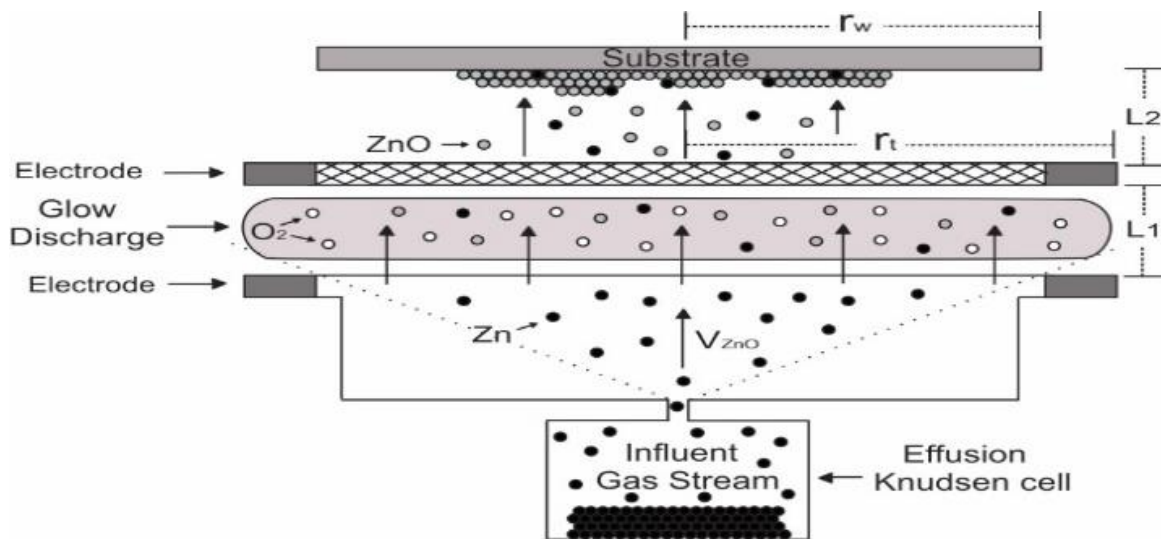
Fig. 1. Représentation schématique du processus d'évaporation réactive assisté par plasma étudié.
