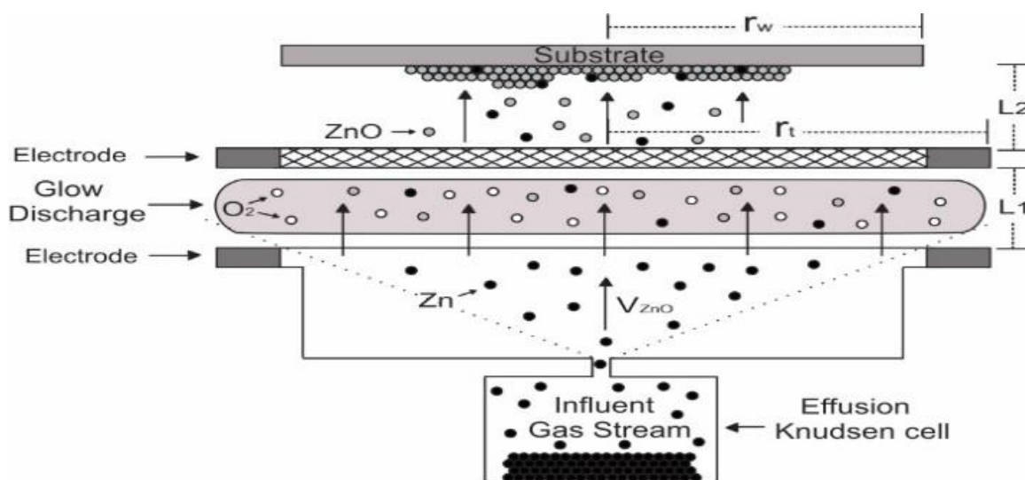
Fig. 1. Représentation schématique du processus d'évaporation réactive assistée par plasma étudié.
