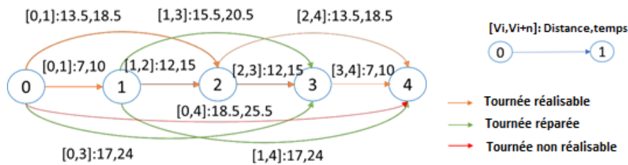
FIGURE 6.3 – SplitGPEVRP - exemple d'un graphe auxiliaire
