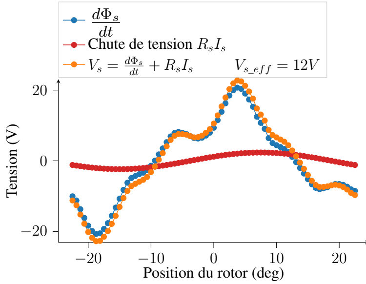
FIGURE 4.7 – Caractéristiques électriques pour le point (190N.m / 200tr.min -1 )
