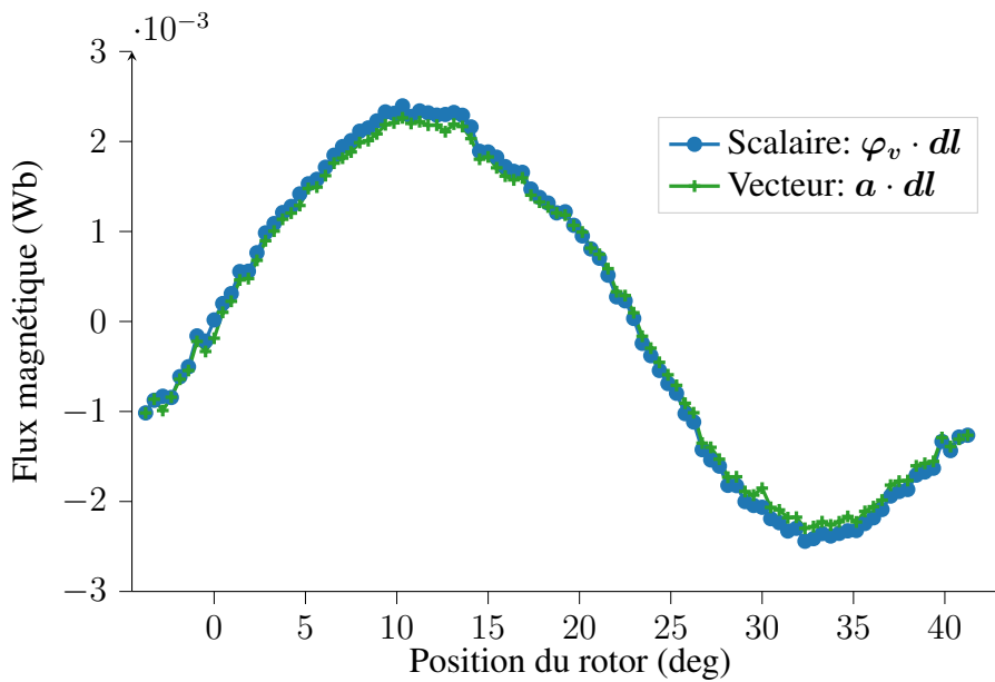
FIGURE 2.6 – Flux calculé sur la MGFA
