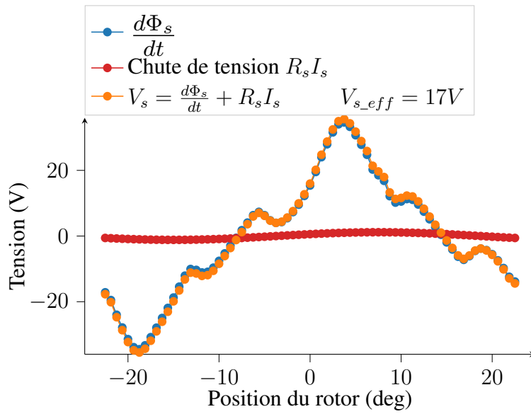
FIGURE 4.8 – Caractéristiques électriques pour le point (77N.m / 500tr.min -1 )
