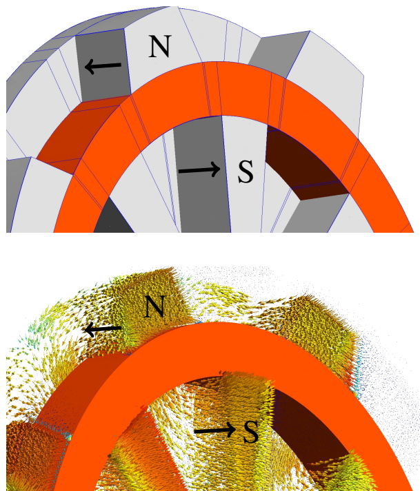
FIGURE 5.4 – Pôles créés par l'inducteur à griffes crampons
