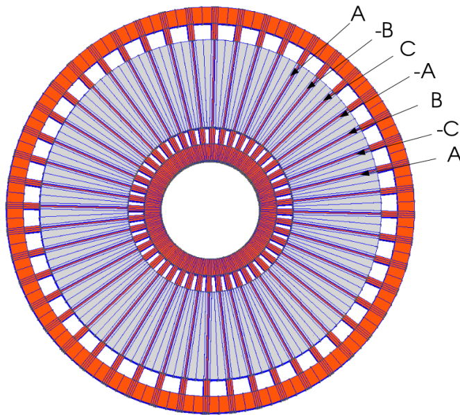
FIGURE 2.11 – Induit initiale : alimentation
