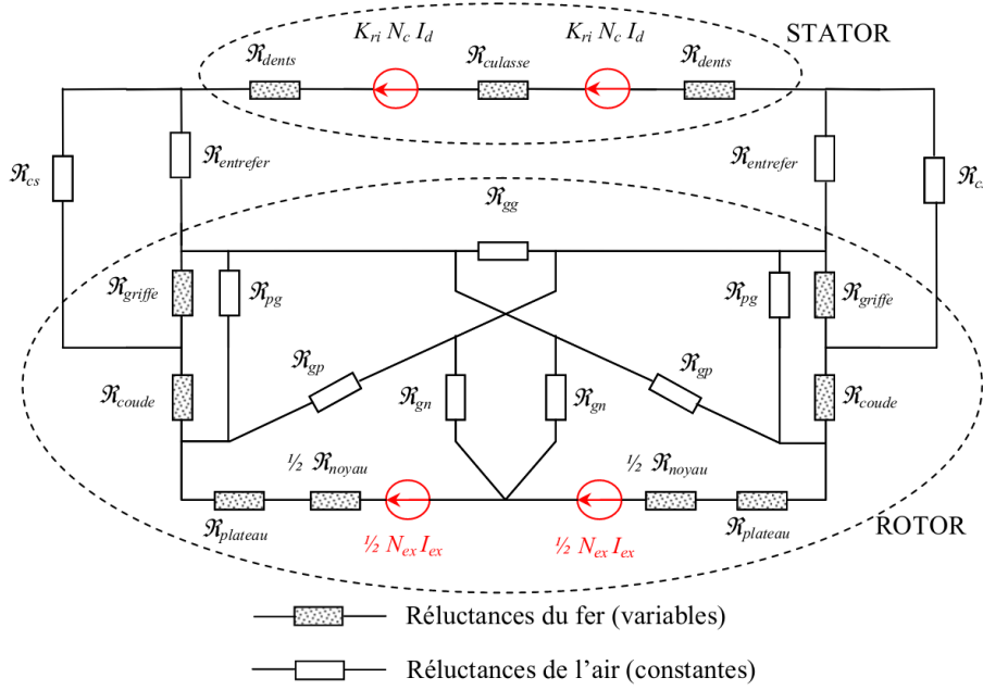
FIGURE 1.9 – Réseau de réductances de L. Albert pour une machine à griffes [Alb04]
