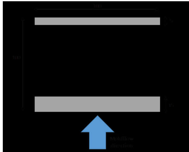
Figure 2.10 : Disposition des éprouvettes découpées pour une orientation des fibres (a) longitudinale (b) intermédiaire et (c) transversale et pour la matrice non renforcée
