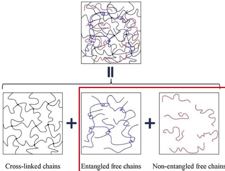
Figure 5.28 : Illustration des différentes interactions entre les chaînes moléculaires susceptibles d'être altérées par l'absorption d'eau [223]
