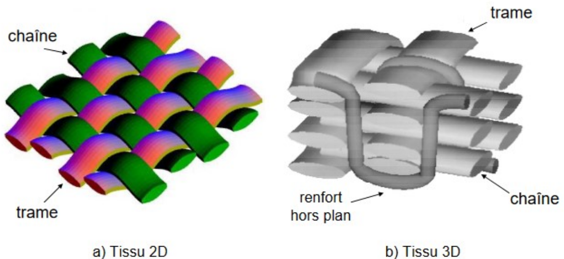
Figure 1.12 : Renforcement tissé avec un tissu a) 2D et b) 3D [40]
