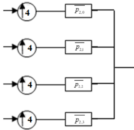
Figure 2.13 Perspective alternative de l'IDWPT pour le multiplexage orthogonal de quatre sous-porteuses [83][84].
