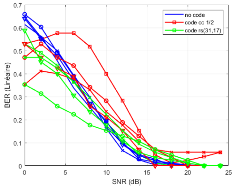
Figure 4.9 BER dans un canal AWGN sans codage, avec codage convolutif et codage Reed Solomon pour 16 utilisateurs en mode MtO
