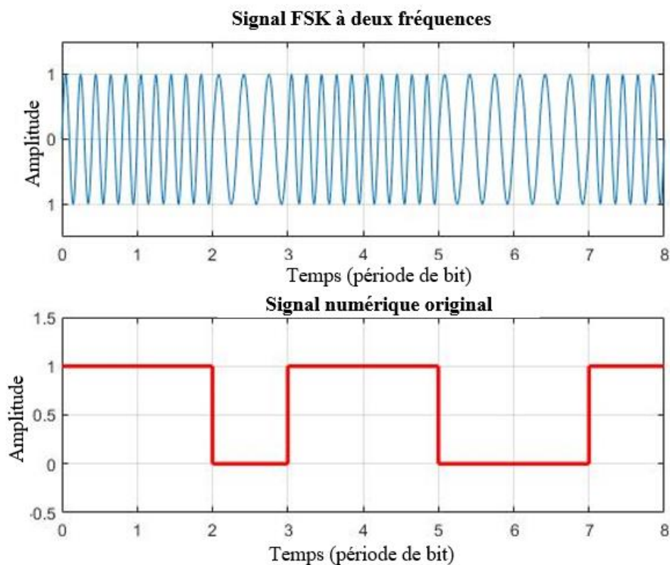
Figure 2.5 La modulation par déplacement de fréquence binaire
