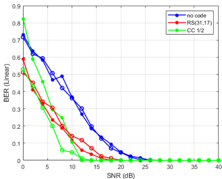
Figure 4.7 BER dans un canal industriel à R=50 sans codage, avec codage convolutif et codage Reed Solomon pour 32 récepteurs en mode OtM
