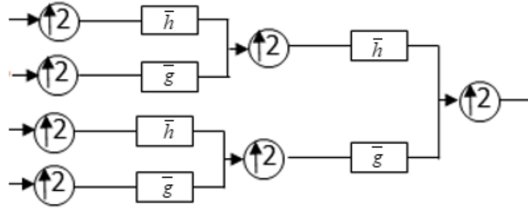
Figure 2.12 Perspective de l'arborescence binaire complète de l'IDWPT pour le multiplexage orthogonal de quatre sous-porteuses [83][84].
