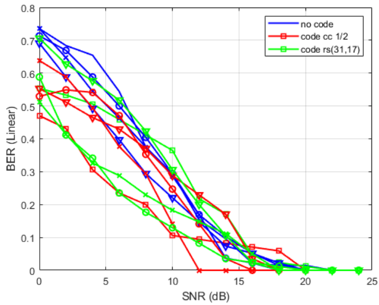
Figure 4.8 BER dans un canal AWGN sans codage, avec codage convolutif et codage Reed Solomon pour 8 utilisateurs en mode MtO
