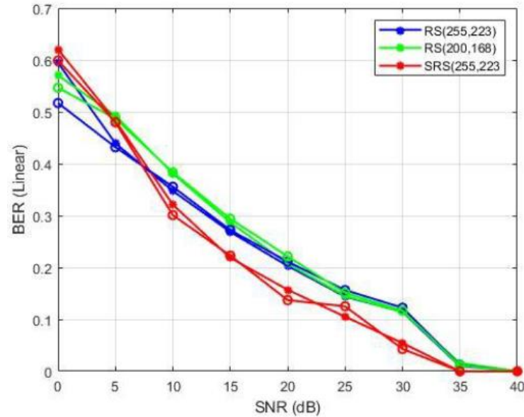
Figure 4.20 Comparaison des performances des différentes combinaison de RS dans un canal AWGN
