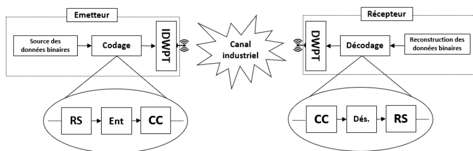
Figure 4.14 Architecture de communication avec combinaison de codage
