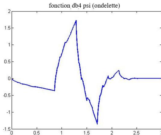
Figure 2.9 Fonction d'ondelettes de Daubechies
