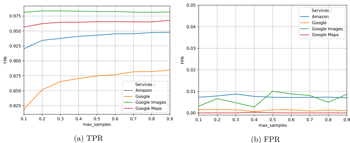
FIGURE 6.4 – Résultats de l'évaluation du paramètre max_samples
