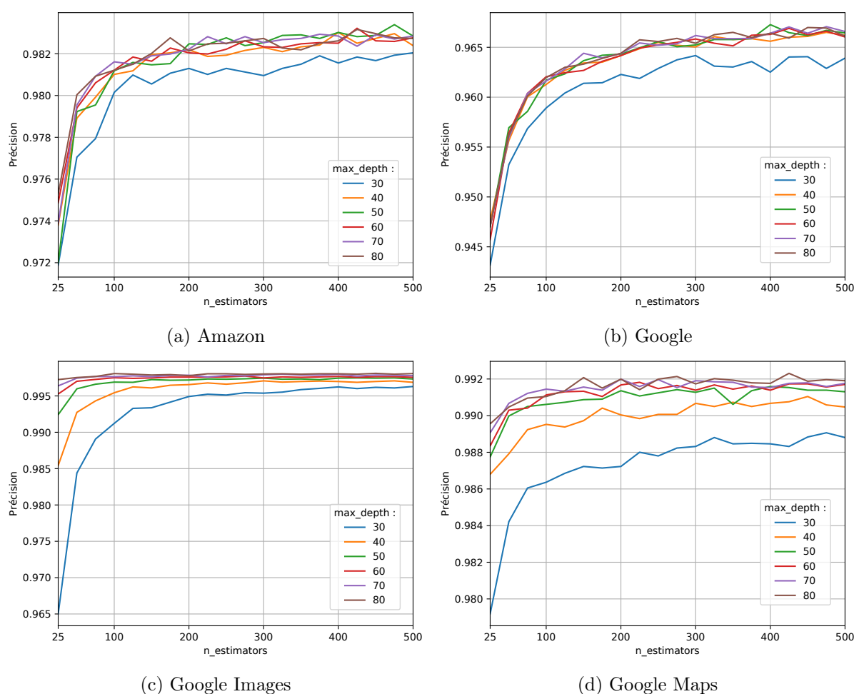
FIGURE 6.1 – TPR pour l'évaluation des paramètres n\_estimators et max\_depth
