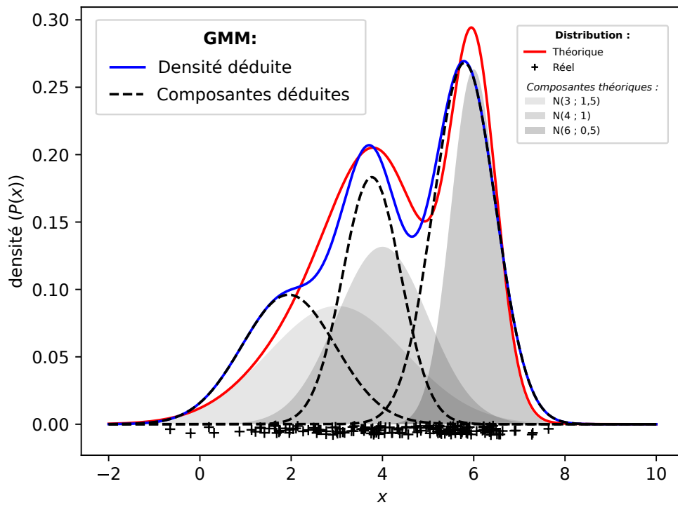
FIGURE 3.5 – Exemple d'application de GMM avec 3 composantes
