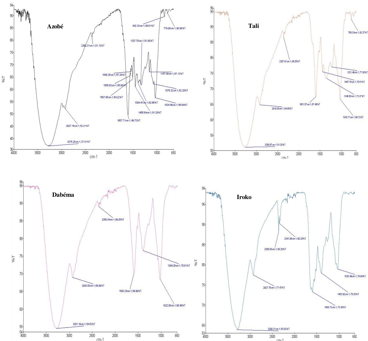
Figure 65 : Spectres FTIR des extraits secs après lyophilisation des écorces extraites par macération à l'eau
