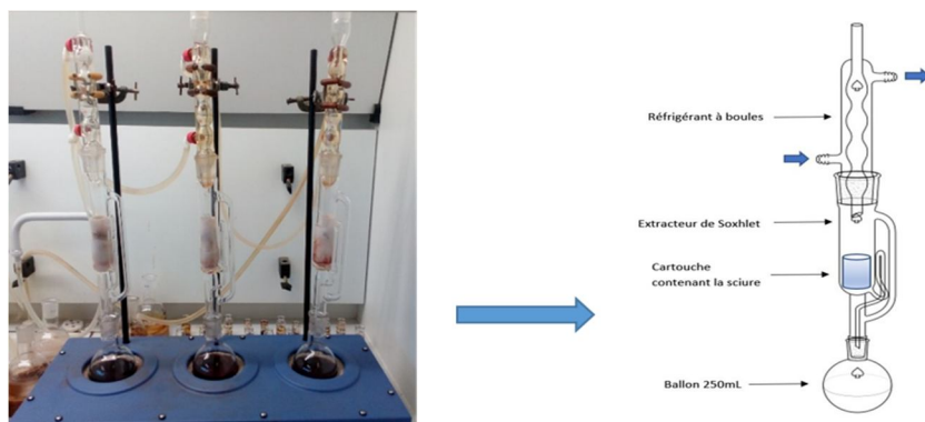
Figure 33 : Dispositif d'extraction au Soxhlet
