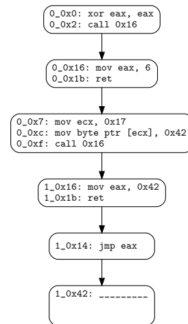
FIGURE 8.1 – Exemple simple d’un code auto-modifiant analysé par BOA
