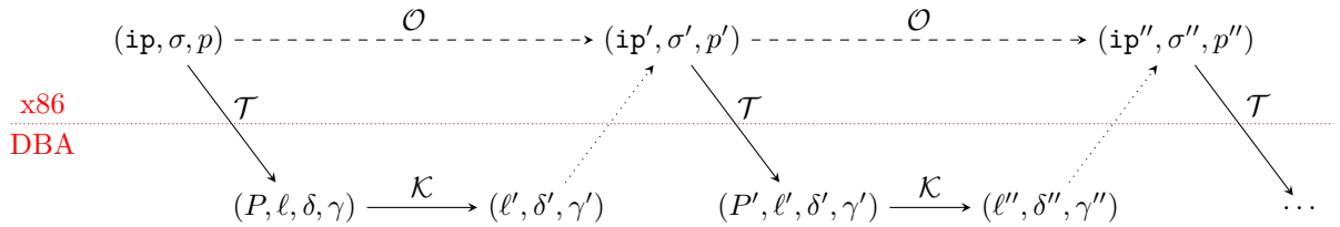
FIGURE 4.1 – Interprétation d'un code binaire x86 via les DBA
