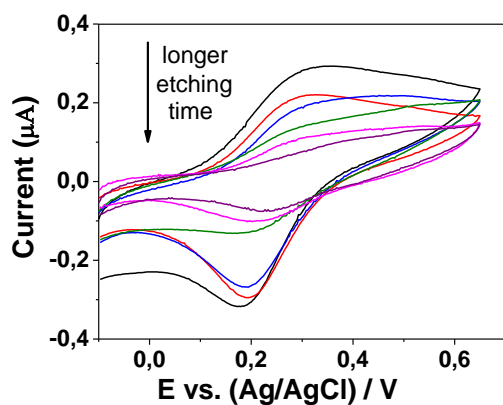
Figure 4 – (A) Évolution du signal électrochimique d'une électrode d'ITO recouverte d'un film de silice mésoporeuse fonctionnalisée par des groupements ferrocène et enregistré dans \text{NaNO}_3 0,1M (vitesse de balayage 5 mV/s) et (B) correspondance entre la variation de l'épaisseur et l'évolution du courant de pic d'oxydation du Fc observée au cours de la réaction avec \text{NH}_4\text{F} 0,05 M
