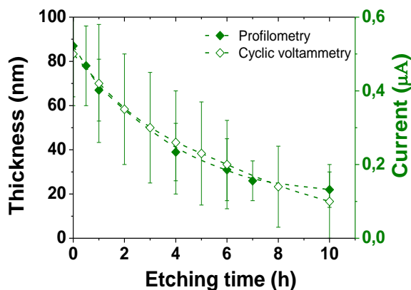
Figure 4 – (A) Évolution du signal électrochimique d'une électrode d'ITO recouverte d'un film de silice mésoporeuse fonctionnalisée par des groupements ferrocène et enregistré dans \text{NaNO}_3 0,1M (vitesse de balayage 5 mV/s) et (B) correspondance entre la variation de l'épaisseur et l'évolution du courant de pic d'oxydation du Fc observée au cours de la réaction avec \text{NH}_4\text{F} 0,05 M
