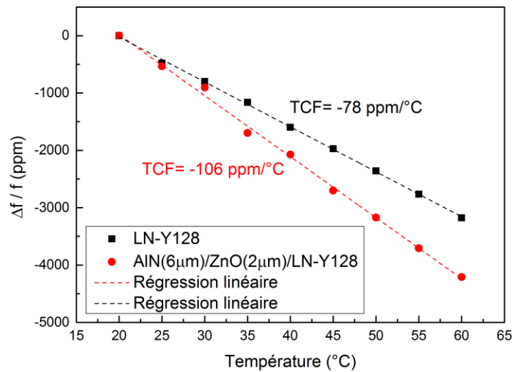
Figure 15 : Coefficient température-fréquence (TCF) du LN-Y128 et de la structure AlN/ZnO/LN-Y128 pour les ondes de type Rayleigh 5
