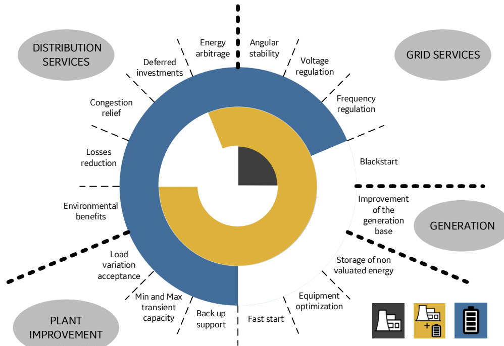
Figure 2.1 : Comparaison des services réalisables par un BESS standalone, une CCGT et une centrale CCGT hybride. Source (F.Kremer et al. , 2019)
