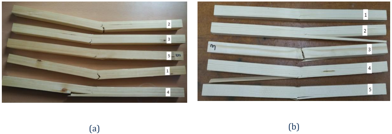
Figure 3.9 : Mode de rupture des éprouvettes de flexion de l'épicéa densifié (a) et de l'épicéa non-densifié (b)
