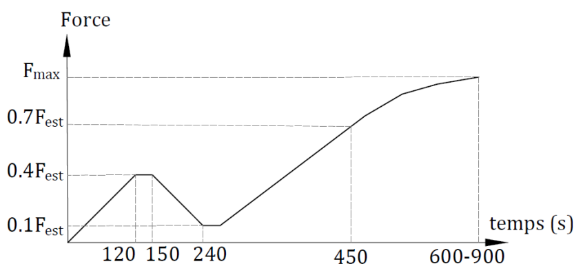
Figure 3.18 : Courbe de chargement des tests de cisaillement double sous des charges monotones [53]
