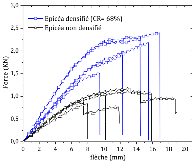
Figure 3.8 : courbes expérimentales force-flèche des tests de flexions 3-points réalisés sur l'épicéa et l'épicéa densifié
