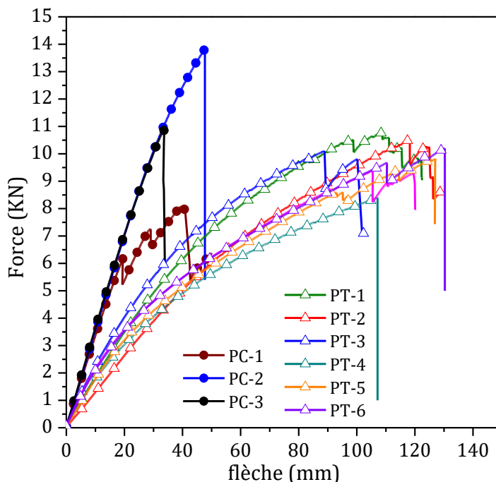
Figure 3.43 : Comparaison des courbes force-flèche des poutres tourillonnées (PT) et des poutres collées (PC)
