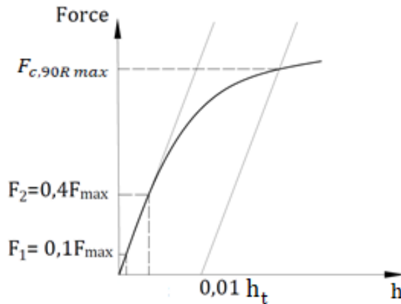
Figure 3.12 : Détermination de la force maximale en compression radiale.
