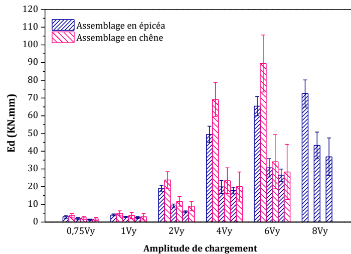
Figure 3.34 : Comparaison des valeurs de l'énergie dissipée des assemblages en épicéa et en chêne pour différents niveaux de chargement
