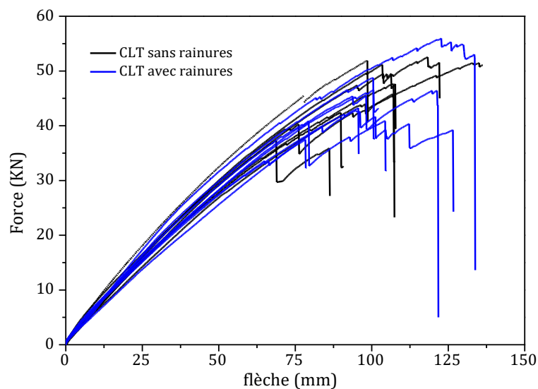
Figure 3.66 : Courbes force-flèche des tests de flexion pour les panneaux CLT avec ou sans rainures
