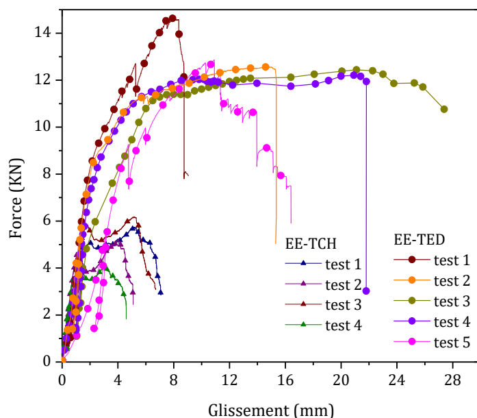
Figure 3.23 : Comparaison des courbes force-glisement des assemblages en épicea
