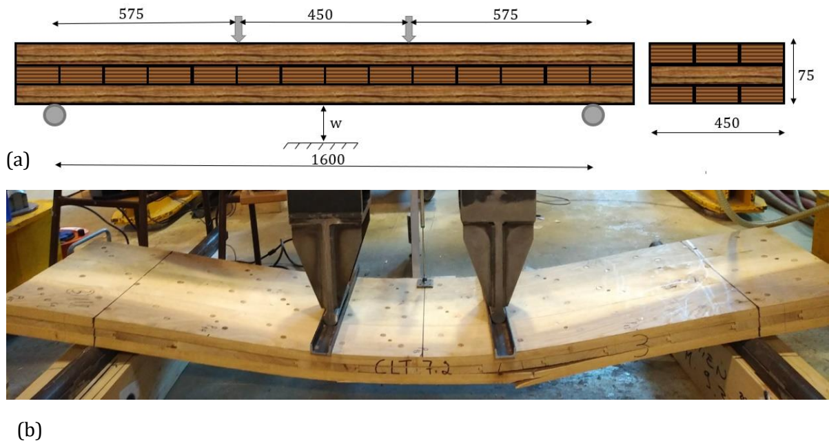
Figure 3.65 : Test de flexion 4-points sur les panneaux CLT : (a) Description géométrique ; (b) Dispositif expérimental
