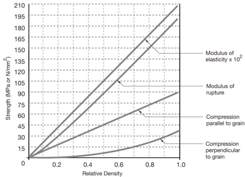
Figure 4.14 : Effet de la densité sur les propriétés mécaniques du bois [CSA O86][99]
