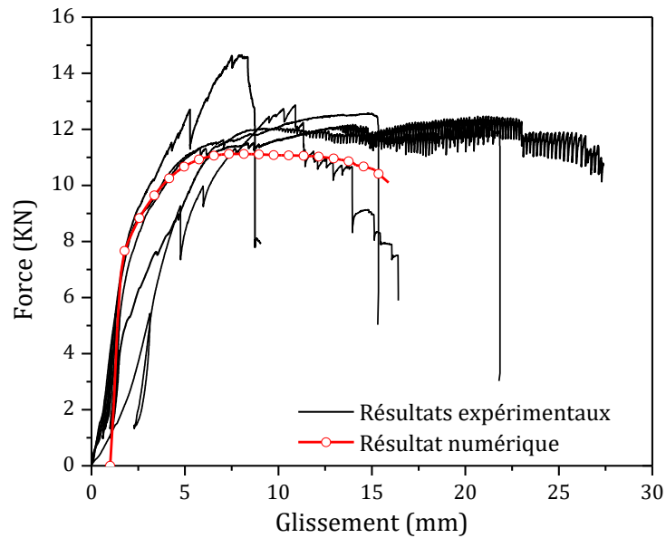
Figure 4.27 : Comparaison des courbes Force-glisserment pour l'assemblage bois/bois
