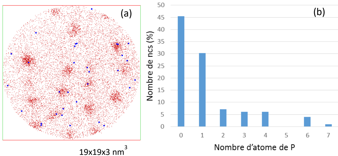
Figure 4.49 : (a) Cartographie atomique sur une vue en coupe de l'échantillon SiO (2,5 nm)/SiO 2 (5,0 nm) préparé avec T cel = 750 °C. Les points rouges et bleus correspondent aux atomes de Si et du P respectivement. (b) Distribution du nombre d'atomes de P comptabilisés dans les nanocristaux de Si.
