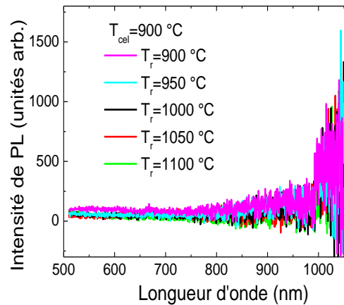
Figure 4.24 : Spectres de photoluminescence pour une multicouche SiO (2,5 nm)/SiO 2 (5,0 nm) préparée avec différentes valeurs de T cel , en fonction de la température de recuit.
