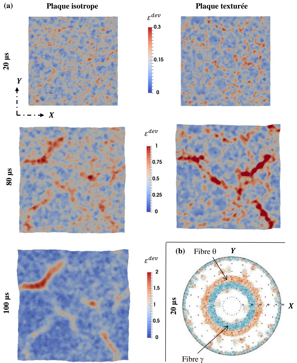
Figure 2.16 : (a) Cartes de la déformation déviatoire \varepsilon^{dev} dans le plan médian pour la plaque de 4000 grains texturée aux temps t = 20 \mu s et 80 \mu s et comparaison avec le cas de la plaque isotrope. (b) carte de la déformation déviatoire \varepsilon^{dev} en projection stéréographique pour la plaque texturée a t = 20 \mu s .
