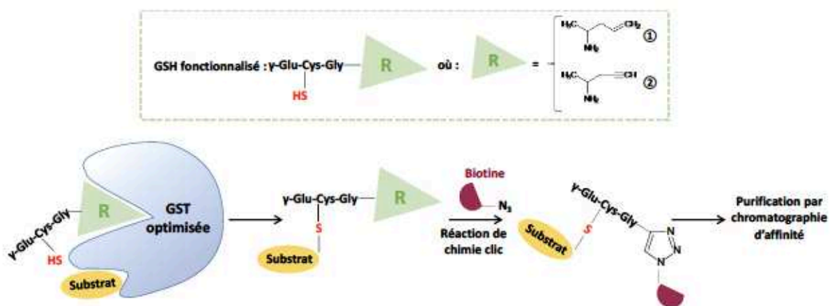
Figure 20 : Principe général de la technique de piégeage in vitro par glutathion (γ-Glu-Cys-Gly) étiqueté (Modifiée de Feng et al. , 2014).
