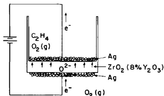
Figure I-7 : Schéma de la cellule électrochimique utilisée pour la première observation du phénomène de la promotion électrochimique de la catalyse [16].
