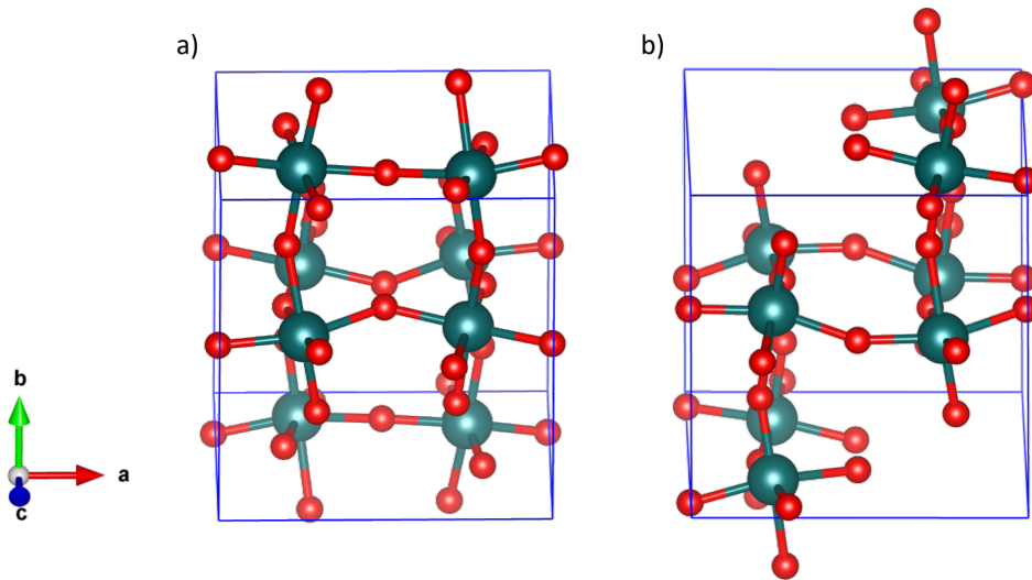
Figure A.2: Structure cristalline relâchée a niveau LDA de la \gamma monoclinique phase (à gauche) et la phase triclinique (à droite) de \text{WO}_3
