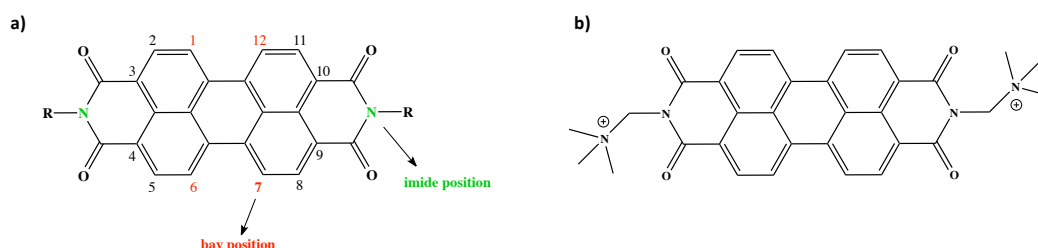
Figure A.1: a) Structure chimique d'un sensibilisateur générique PDI: les positions de la baie et de l'imide sont indiquées respectivement en rouge et en vert. b) Molécule de bis-imide PDI d'acide N,N'-bis(2-(triméthylammonium)-éthylène)-pérylène-3,4,9,10 tétracarboxylique étudiée dans cette thèse.
