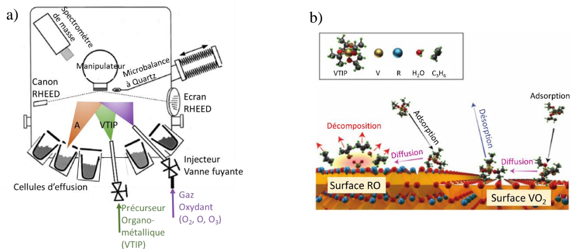
Figure 40 : a) Schéma de conception d'une enceinte MBE hybride avec un injecteur de gaz oxydant (O 2 , O, O 3 ...) et un injecteur d'un précurseur gazeux (VTIP, TTIP ...). Les autres éléments de l'enceinte sont ceux d'une MBE standard. b) Schéma des mécanismes de croissance avec un précurseur VTIP sur une surface de RVO 3 . L'intégration de VO 2 à la surface est sélective et nécessite une surface RO. (Adapté de [110]).
