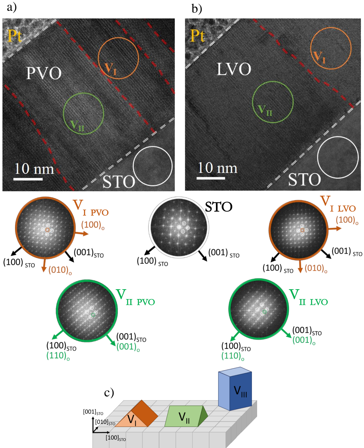
Figure 89 : Observations TEM de films optimisés de PVO a) et LVO b). L'observation est effectuée selon l'axe de zone [010] STO. Les interfaces avec le substrat et le Pt de protection sont indiquées par les pointillés blancs. La présence de variants V I et V II est indiquée par les cercles oranges et verts respectivement. Le substrat est indiqué par le cercle blanc. En c) une représentation de ces variants est donnée en rappel. En a) et b) les interfaces entre variants sont indiquées en pointillés rouges. La détermination des variants se fait par l'observations des FFT. Celles-ci sont données pour le STO (cercle blanc) et les deux variants dans leur couleur respective. La correspondance des directions orthorhombiques et les pics de diffraction supplémentaires sont également indiqués dans leur couleur respective.
