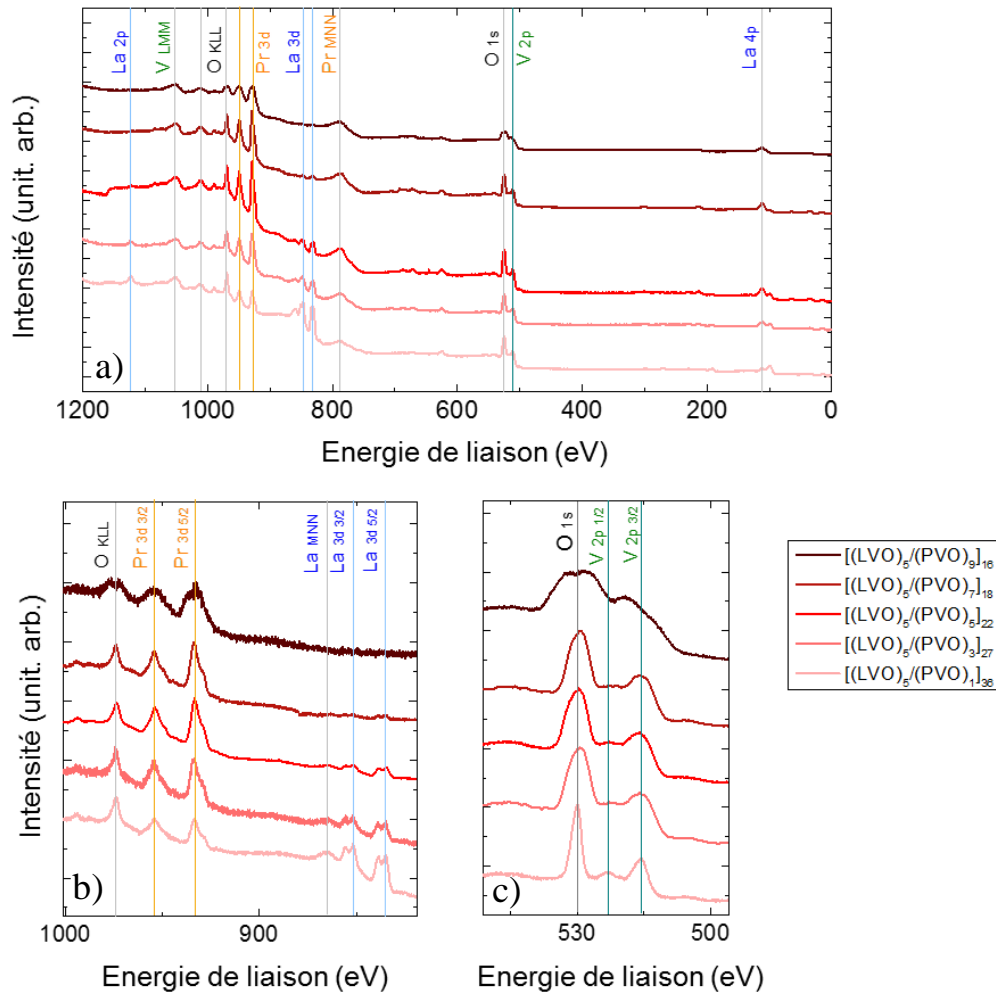
Figure 121 : Profils XPS des superréseaux [(LVO) 5 /(PVO) n ] in situ . Mesures faites avec une électrode Al non monochromatique de raie principale K \alpha -1 = 1486,7 eV. L'angle d'incidence est d'environ 45°. Les mesures sont faites avec un détecteur hémisphérique. Spectres d'ensemble en a) et spectres autour des seuils de Pr 3d et V2p respectivement en b) et c). L'évolution de l'intensité des pics de La 3d est également visible en b) avec le changement de motif.
