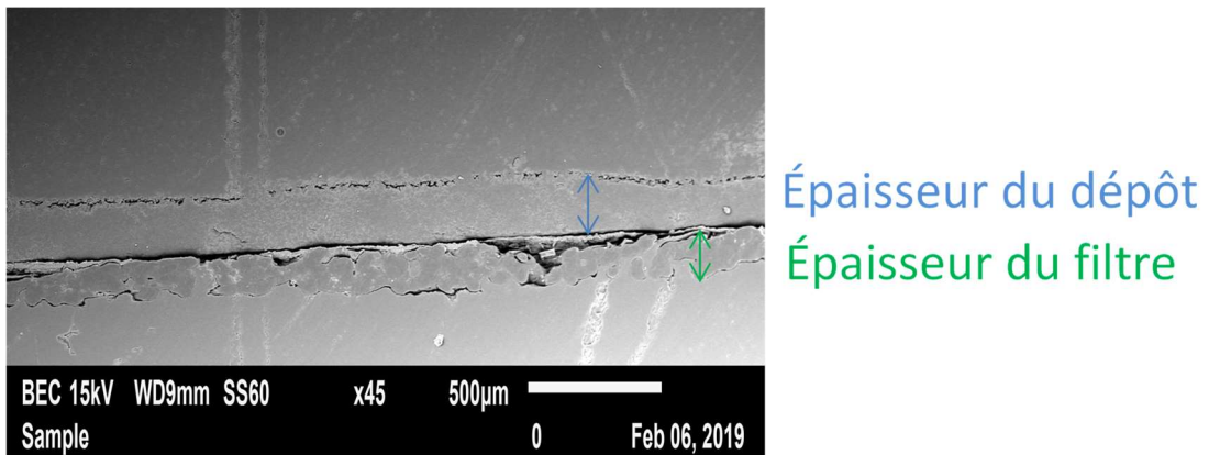
Figure 62 : Image MEB d'une vue large d'un dépôt de nanoparticules de KCl mis sous résine
