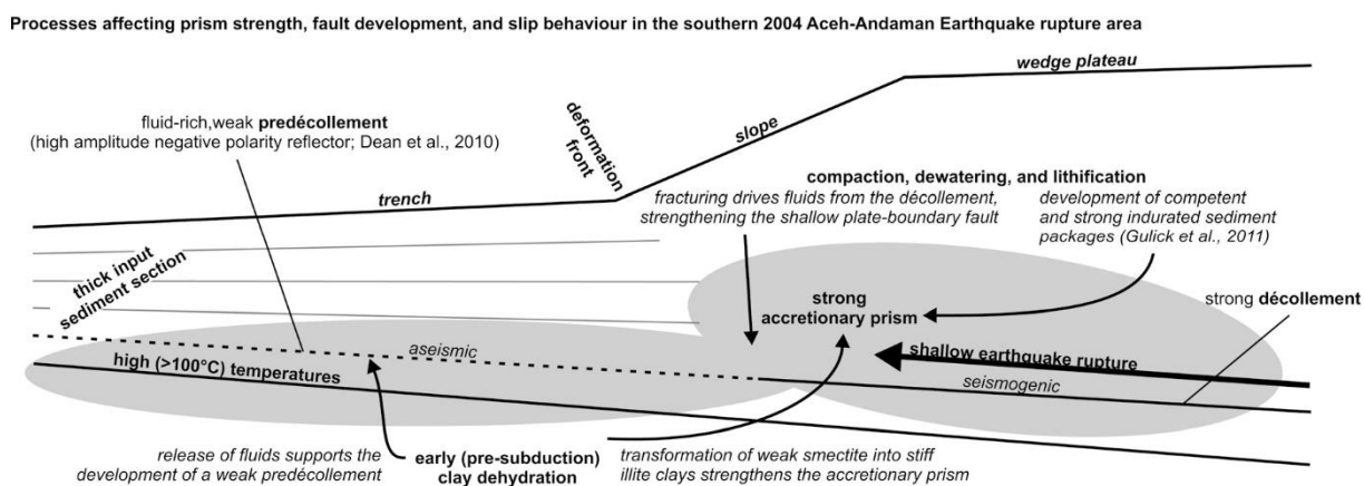
Figure 34 : Synthèse des processus physiques, diagénétiques et hydrogéologiques impliqués dans la rupture sismogène et tsunamigène de l'interface de subduction à faible profondeur de la marge nord de Sumatra, déduits des études géophysiques préalables à l'expédition IODP 362 (Geersen et al., 2013).
