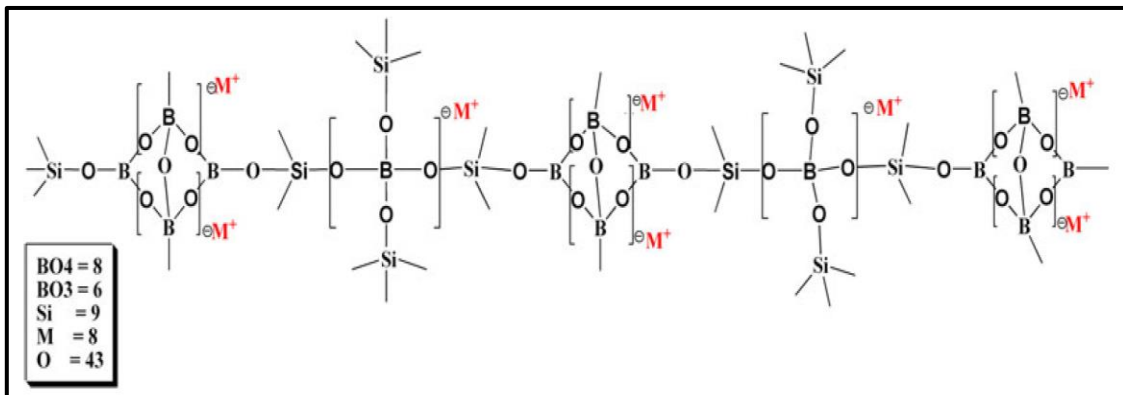
Figure 12 : Unité de base du verre à quatre éléments (\text{SiO}_2)_{0,45} (\text{B}_2\text{O}_3)_{0,35} (\text{Na}_2\text{O})_{0,175} (\text{Cs}_2\text{O})_{0,025}
