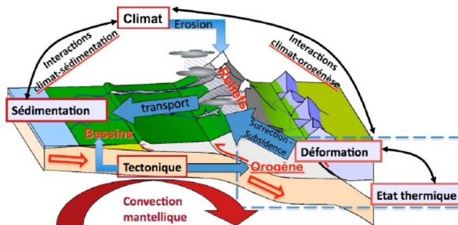
FIGURE 1.4 – Schématisation des interactions entre la géologie, le climat et l'hydrologie ( http://lgltp.ens-lyon.fr/recherche/surface-et-lithosphere ).
