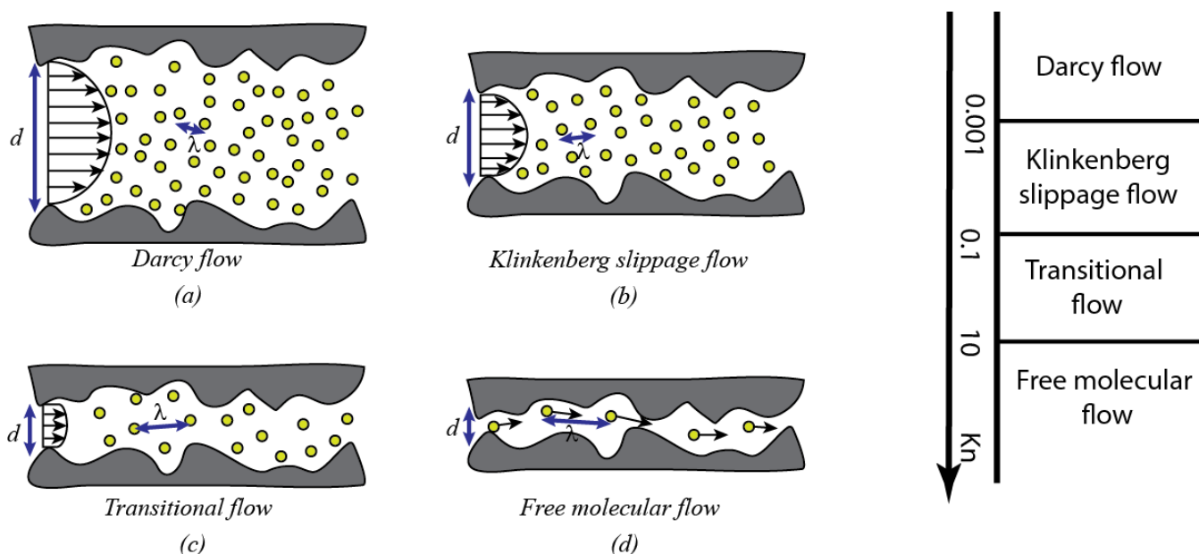
Fig.2: Les différents régimes de transfert de gaz dans les milieux poreux non-conventionnel selon les gammes de nombre de Knudsen
