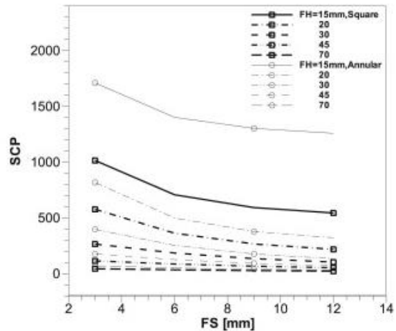
fig. 18 SCP avec lit identique
