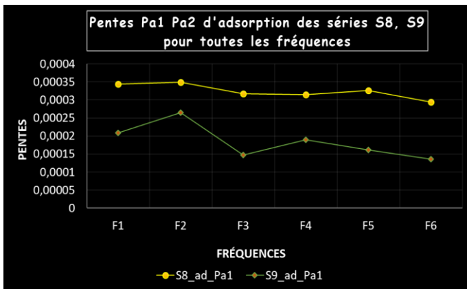
fig. 65 : Pentas d'adsorption Série S8, S9
