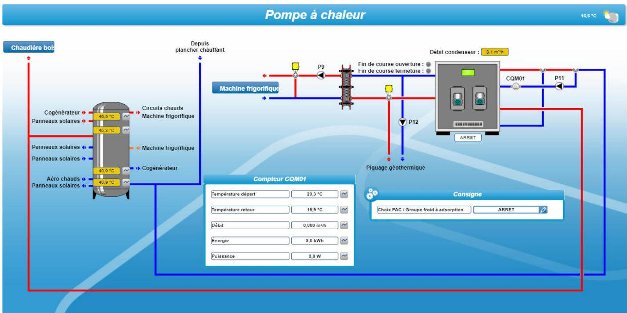
fig. 179 : Pompe à chaleur
