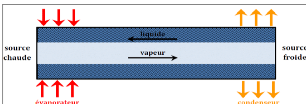
fig. 85: principe de fonctionnement d'un caloduc
