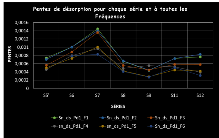
fig. 74: Evolution des pentes de désorptions pour toutes les fréquences en fonction des séries
