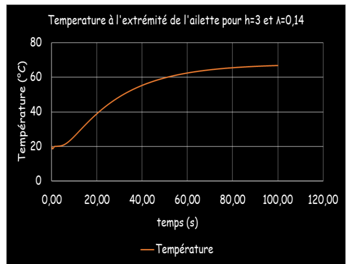
fig. 149: Profil de température à l'extrémité de l'ailette en fonction du temps.
