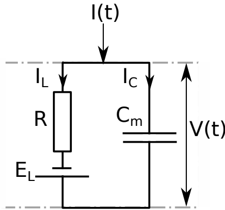
Fig. 1.4 – Représentation de l'activité neuronale du modèle LIF par un circuit électrique.
