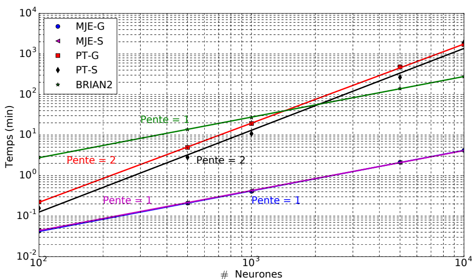
Fig. 2.6 – Le temps d’exécution est comparé en fonction de la taille d’un réseau MSN avec 30% de connectivité pour différentes approches de simulation, PT-S, PT-G, MJE-S, MJE-E et le simulateur BRIAN2. . Tirée de l’article [13].
