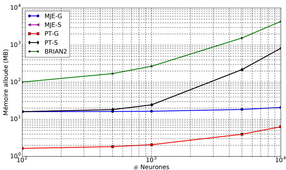
Fig. 2.7 – La mémoire allouée est comparée en fonction de la taille d’un réseau MSN avec 30% de connectivité pour différentes approches de simulation, PT-S, PT-G, MJE-S, MJE-E et le simulateur BRIAN2, tirée de l’article [13].
