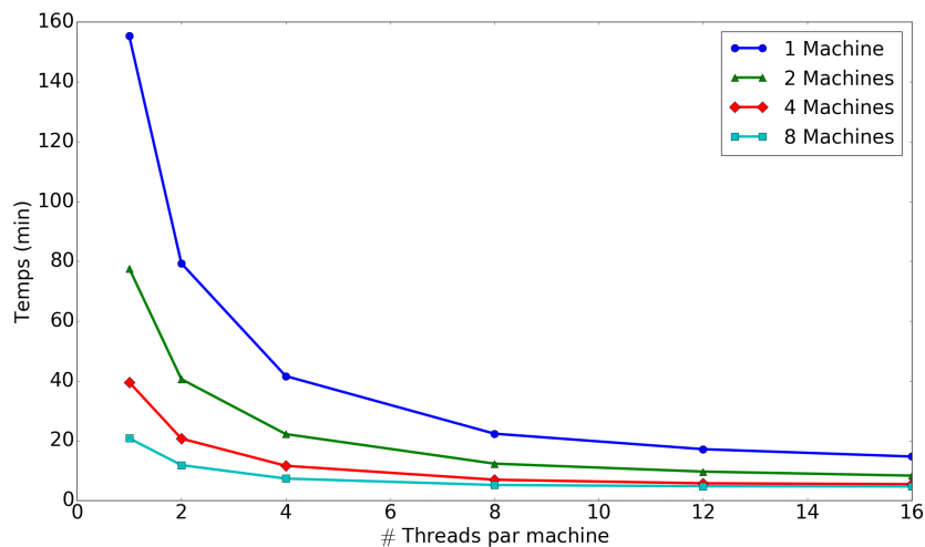
Fig. 3.19 – Temps d'exécution en fonction du nombre de threads avec la méthode MTMM pour la simulation d'un réseau MSN avec 100 000 neurones, et 504 connexions entrantes par neurone, pendant 1s de temps biologique.
