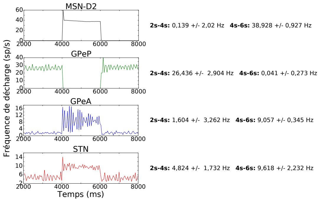
Fig. 5.6 – Fréquences de décharge du réseau lors d’une excitation du MSN-D2.
