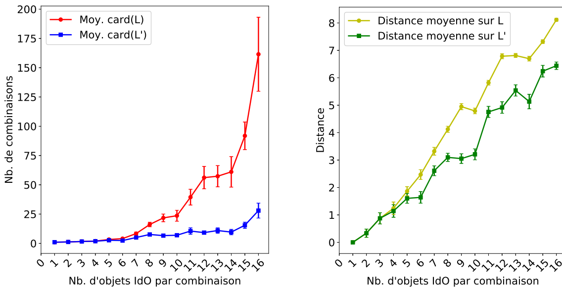
(a) Nb. moyen de combinaisons d'actions trouvées dans les listes L et L' selon le nombre d'objets IdO concernés par une combinaison. L'intervalle de confiance est configuré à 68%. (b) Distance moyenne des combinaisons d'actions trouvées dans les listes L et L' selon le nombre d'objets IdO concernés par une combinaison. L'intervalle de confiance est configuré à 68%.
