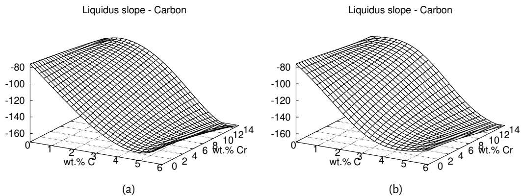
Fig. 8 - Rapport de la pente de liquidus données par la régression avec le modèle AMN-MLP à la pente de liquidus calculée par le logiciel Thermo-Calc® à gauche pour le carbone, à droite pour le chrome
