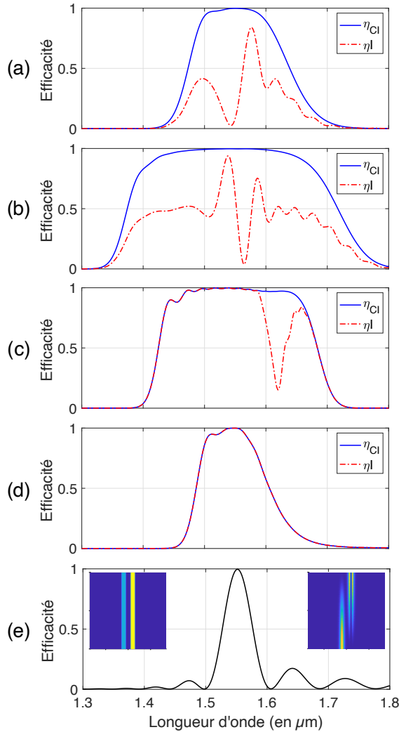
FIGURE 4.6 – (a), (b), (c), (d), (e) Évolution de \eta_{C1} (courbe bleue continue) et \eta_l (courbe pointillée rouge) en fonction de \lambda pour différents convertisseurs adiabatiques du mode 0 ( \alpha_i = 1 ) au mode 1 ( \alpha_o = 2.40 ) dont l'évolution en z a été étudié à \lambda = 1.55 \mu\text{m} sur la Fig. 4.4 : (a) \alpha_2 = 1 (STIRAP sur le mode 0 dans WG2 à \lambda = 1.55 \mu\text{m} avec la propagation correspondante dans la Fig. 4.4 (a)), (b) \alpha_2 = 2.4 (STIRAP sur le mode 1 dans WG2 à \lambda = 1.55 \mu\text{m} , Fig. 4.4 (b)), (c) \alpha_2 = 5.6 (Fig. 4.4 (c) à \lambda = 1.55 \mu\text{m} ), (d) \alpha_2 = 7 (Fig. 4.4 (d) à \lambda = 1.55 \mu\text{m} ). (e) Comparaison avec la bande passante d'un convertisseur de mode 01 basé sur un coupleur directionnel. La structures des deux guides droits est donnée dans l'encart à gauche ( L = 8 \text{ mm} et s_0 = W , les autres paramètres restent inchangés) et celui de droite illustre la propagation à \lambda = 1.55 \mu\text{m} .
