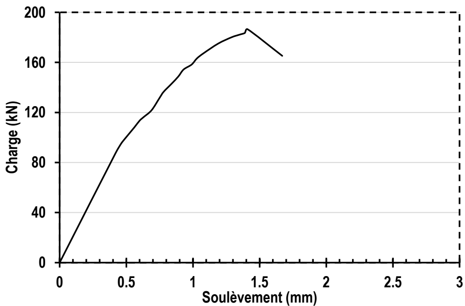
(b) Courbe charge-soulèvement des connecteurs 'OCAL-(3x50)'.
