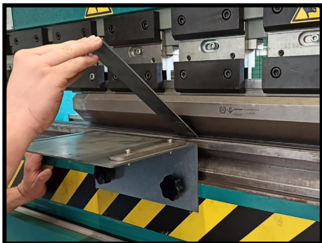
(c) Pliages pour former les deux montants latéraux du connecteur OMEGA.
