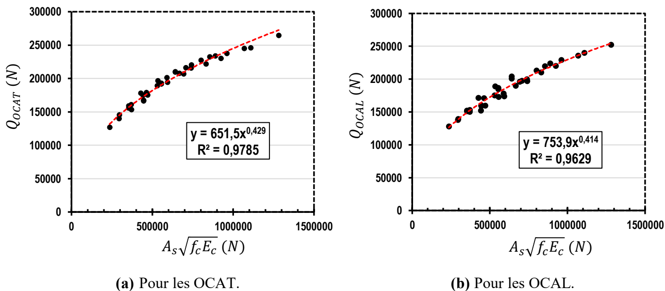
Figure 4.22 Développement de la formule de résistance des connecteurs OMEGA par ligne de tendance.
