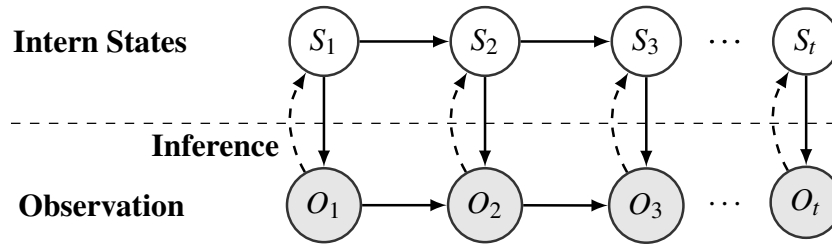
FIGURE 3.11 – Processus d'inférence
