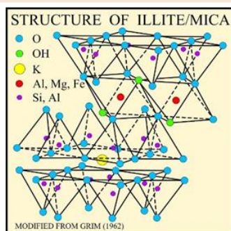
Structure des feuillets de l'illite (Poppe et al., 2001)
