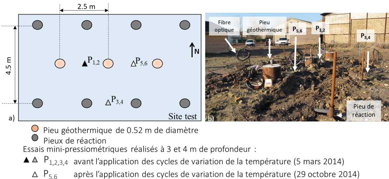
Figure II. 58 : a) Plan de localisation des pieux géothermiques et des essais mini-pressiométriques réalisés ; b) Photographie du site instrumenté.
