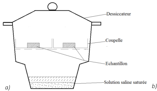
Figure II. 70 : a) Schéma de principe d'imposition de la succion par phase vapeur ; b) Relation entre l'humidité relative et la succion imposée en fonction de la nature du sel
