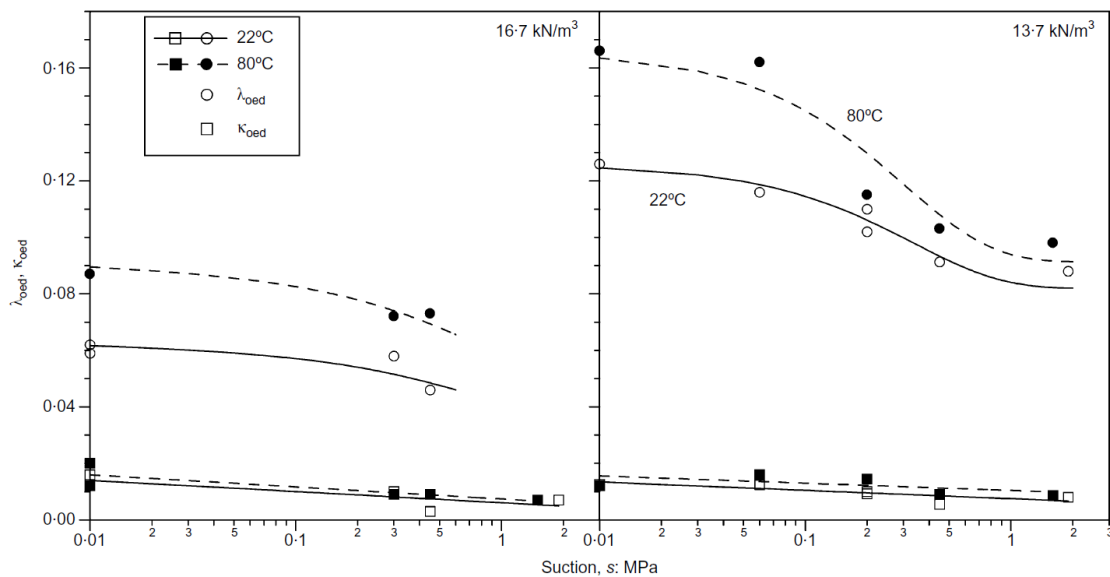
Figure II. 19 : Variation en fonction de la température du coefficient \kappa_{oed} caractérisant la déformation élastique pré-seuil d'un essai œdométrique et \lambda_{oed} caractérisant la déformation plastique post-seuil pour des essais de compressibilité réalisés sous différentes succions et deux températures (Romero et al. 2003). Les essais ont été réalisés sur des éprouvettes préparées à deux densité ( \gamma_d = 16,7 et 13,7 \text{ kN/m}^3 )
