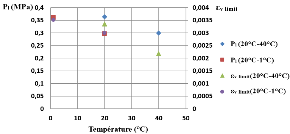
Figure II. 56 : Variation de la pression limite P_i et de la déformation limite \epsilon_{v \text{ limit}} en fonction de la température.
