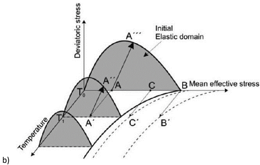
Figure II. 6 : a) Cadre théorique schématisé de l'évolution de la limite entre le domaine élastique en grisé et le domaine pseudo-élastique des sols chauffés (Laloui et Di Dona 2013) dans le plan contrainte effective moyenne-température et b) son extension en trois dimensions en considérant la contrainte déviatorique.
