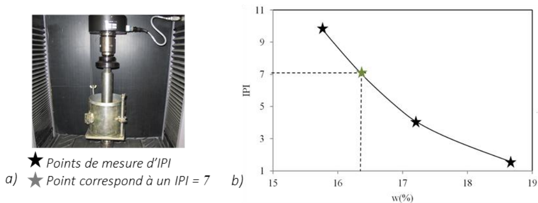
Figure II. 74 : a) Essai de poinçonnement, b) Variation de l'IPI sur les points de la courbe Proctor du limon LP.
