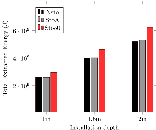
Figure II. 93 : Comparaison de Energie Totale extraite (TEE) entre les scénarios de stockage de la chaleur (StoA et Sto50), et le scénario sans stockage (NSto) à trois profondeurs d'installation différentes.
