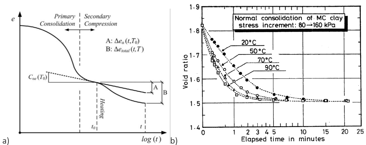
Figure II. 30 : a) Représentation schématique de la courbe de consolidation lors de l'application d'une contrainte mécanique puis thermomécanique (Coccia et McCartney, 2016). b) Effet de la température sur le taux de consolidation d'une argile normalement consolidée (Towhata et al. 1993).
