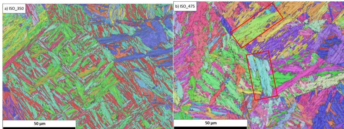
Figure 3 : Cartographie EBSD de l'indice de qualité et l'IPF des phases ferritiques après traitements isothermes à a) 350 °C et b) 475 °C. Les cadres rouges permettent d'identifier des paquets contenant un seul variant bainitique.
