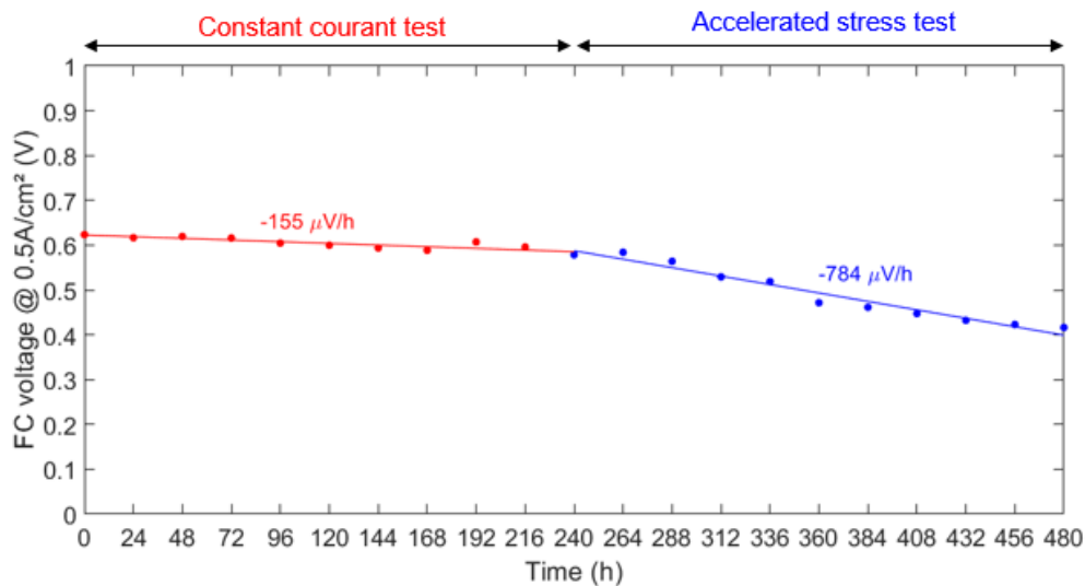
Figure 2.2 : Évolution de la tension de cellule à 0,5 \text{ A/cm}^2 pendant 240 h de fonctionnement à courant constant ( 0,5 \text{ A/cm}^2 ) suivi de 240 h d'AST réalisé avec un AME avec un manque de couche active près de l'entrée de l'anode et deux défauts d'induction, à l'anode également. Les taux de dégradation de la tension ont été estimés par interpolation linéaire.
