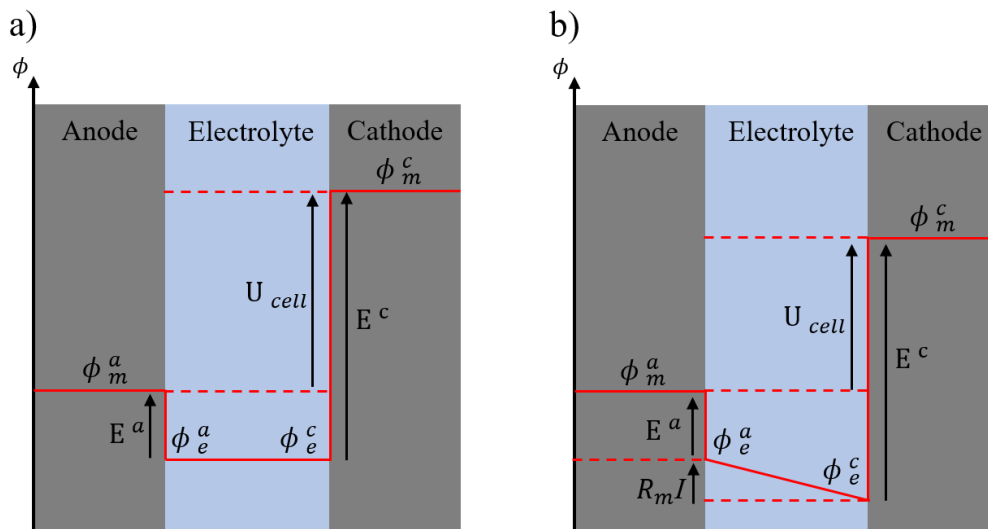
Figure 2.18 : Représentation des potentiels cathodique et anodique en fonction des potentiels de la phase métallique et de la phase ionique ; a) en absence et b) en présence de courant. Adapté de la référence [123].
