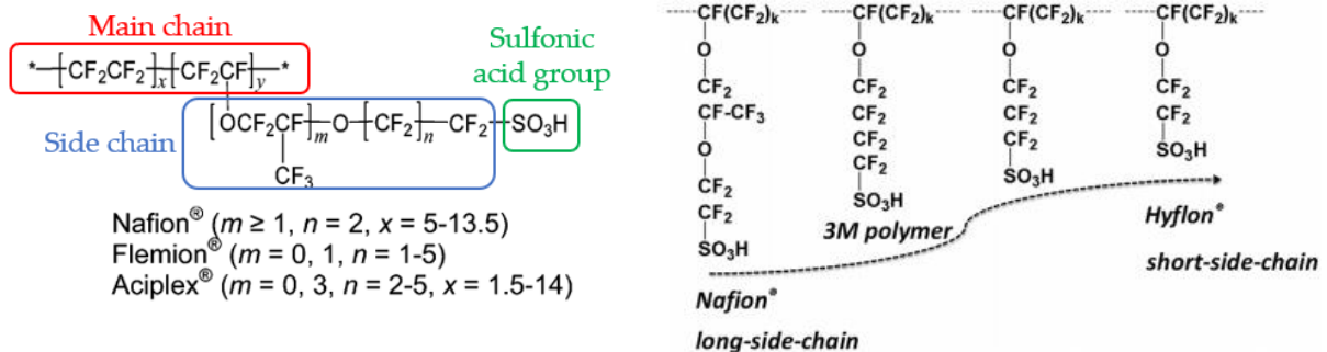
Figure 1.16 : À gauche : Structures chimiques des membranes à électrolyte polymère ayant des chaînes latérales longues (ex. : Nafion®, Flemion® et Aciplex®). À droite : Diverses structures de ionomères PFSA. Les figures sont adaptées des références [114,157].
