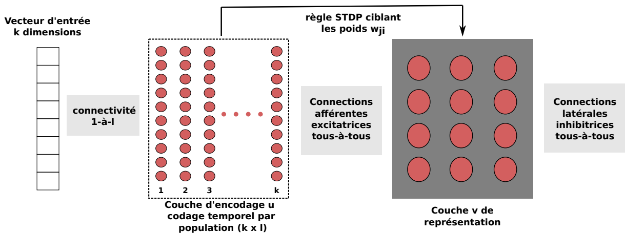
FIGURE 4.1 – Schéma bloc de l'architecture du SNN. Soit un vecteur d'entrée à k dimensions. Une dimension du vecteur d'entrée est encodée par l neurones. L'activité éparse des k \times l neurones est transmise à la couche de représentation. Entre ces deux couches s'opère l'apprentissage des poids synaptiques w_{ji} avec une nouvelle règle STDP. Des connexions latérales inhibitrices sont présentes dans la couche de représentation pour mettre les neurones en compétition, générant un apprentissage compétitif.
