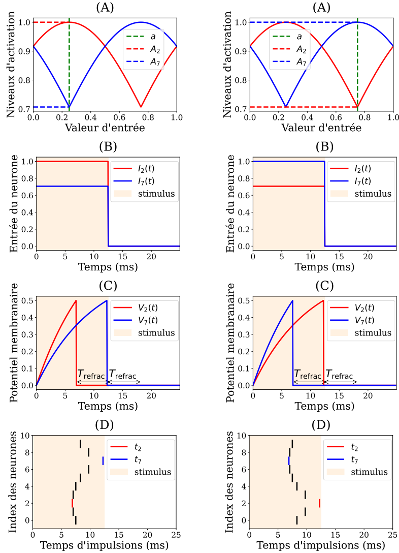
FIGURE 3.3 – Illustration d'un cas de translation spatiale d'un motif impulsionnel. La première et la seconde colonne illustrent l'encodage neuronal d'une entrée a = 0.25 et d'une autre entrée a = 0.75 , respectivement. La rangée (A) montre que le neurone 2 a un champ récepteur centré sur \mu_2 = 0.25 , tandis que le neurone 7 a un champ récepteur centré sur \mu_7 = 0.75 . La valeur des niveaux d'activations A_2 et A_7 est inversée quand on passe d'une valeur d'entrée a = 0.25 à a = 0.75 . L'inversion des niveaux d'activations A_2 et A_7 est due à l'inversion des distances entre les entrées a = 0.25 et a = 0.75 , et les centres \mu_2 = 0.25 et \mu_7 = 0.75 . (C) L'inversion des niveaux d'activations A_2 et A_7 se répercute à son tour par l'inversion de la trajectoire des potentiels membranaires V_2(t) et V_7(t) . (D) Le résultat final est que la structure des temps de décharge représentant l'entrée a = 0.25 est la même que pour a = 0.75 , dans le sens où cette structure a uniquement subi une opération de translation spatiale. Cette translation spatiale est due à la symétrie au centre des gaussiennes, ainsi qu'à l'espace circulaire empêchant les effets de bords (i.e. coupure de la gaussienne). De façon générique, toute translation d'une valeur d'entrée a par un multiple k de 1/l avec l étant le nombre de neurones, génère une translation spatiale du motif impulsionnel représentant a . Plus formellement, si on considère une valeur continue a \in [0, 1] transformée en un motif impulsionnel \mathbf{t} \in [0, T]^l , alors toute valeur a' \in (a \pm k/l) \bmod 1 induit un motif impulsionnel \mathbf{t}' \in [0, T]^l qui est une translation spatiale de \mathbf{t} \in [0, T]^l .
