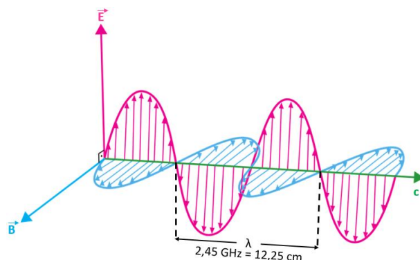
Figure 1. 27 : Représentation d'une onde micro-ondes composée d'un champ électrique (en rose) et d'un champ magnétique (en bleu). c représente la vitesse de la lumière (en vert).
