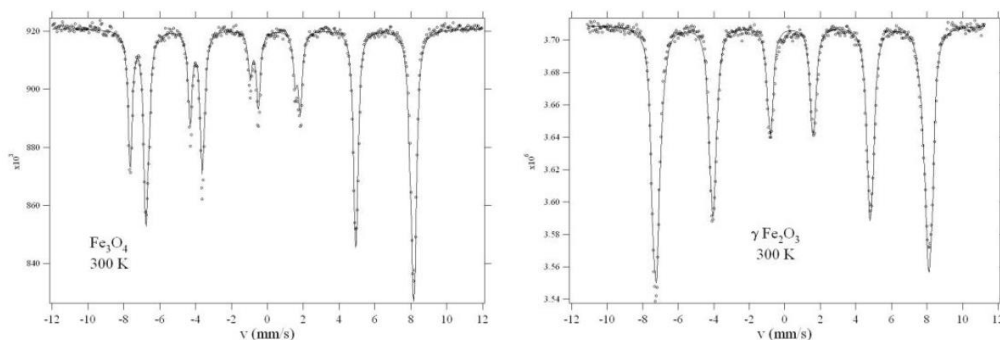
Figure 1. 5: Spectres Mössbauer de la magnétite Fe_3O_4 massive (gauche) et de la maghémite \gamma-Fe_2O_3 massive (droite) à température ambiante [10].
