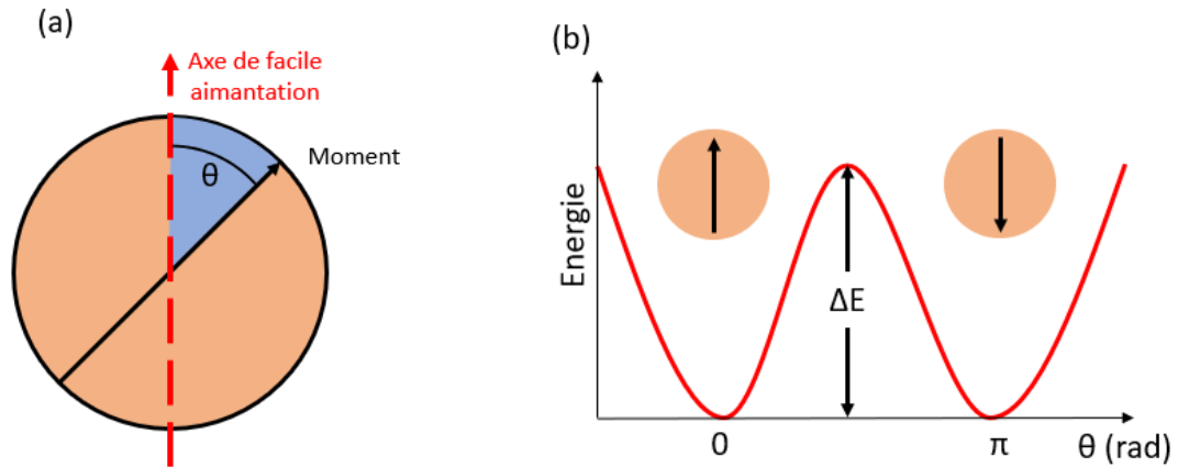
Figure 1.12 : Représentation schématique du vecteur d'aimantation dans une particule mono-domaine dévié d'un angle \theta par rapport à l'axe de facile aimantation (a). Description de l'énergie d'anisotropie magnétocristalline d'une particule mono-domaine en fonction de l'angle \theta entre le moment d'aimantation et l'axe de facile aimantation (b).
