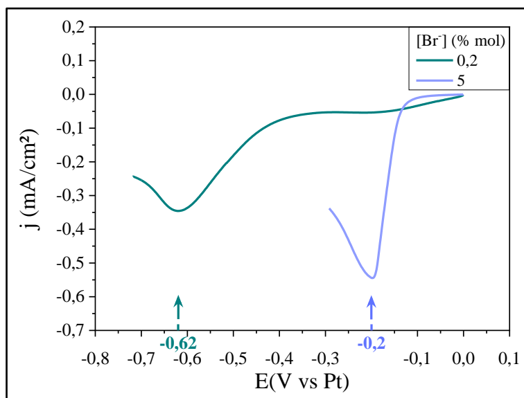
Figure 2.7 : Voltampérogrammes linéaires de Te(IV) obtenus pour des électrolytes EOPipTFSI : EOPipBr 95 : 5 % mol, à 100 °C, 5 mV/s, électrode de travail de Pt, ([Te(IV)] = 5 mM) à différentes concentrations en Br - précisant les potentiels appliqués dans chaque cas pour l'électrodéposition de Te.
