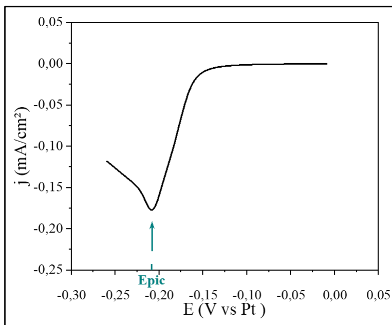
Figure 2.5 : Détermination du potentiel de réduction du Te(IV) par voltampérométrie linéaire : Voltampérogramme type obtenu avec EOPIpTFSI : EOPIpBr 5 %mol, à 100 °C, 5 mV/s, électrode de travail de Pt, [Te(IV)] = 5 mM.
