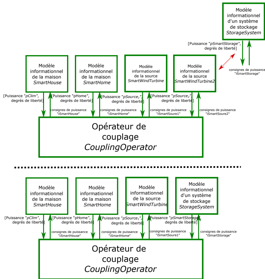
FIGURE 6.11 – Modification d'un composant au multi-modèle 6.10 (source par système de stockage).
