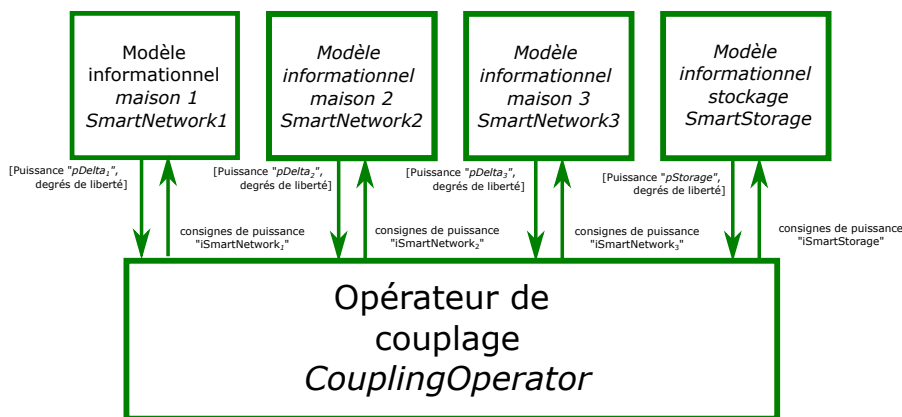
FIGURE 6.18 – Multi-modèle de micro-réseau construit hiérarchiquement.
