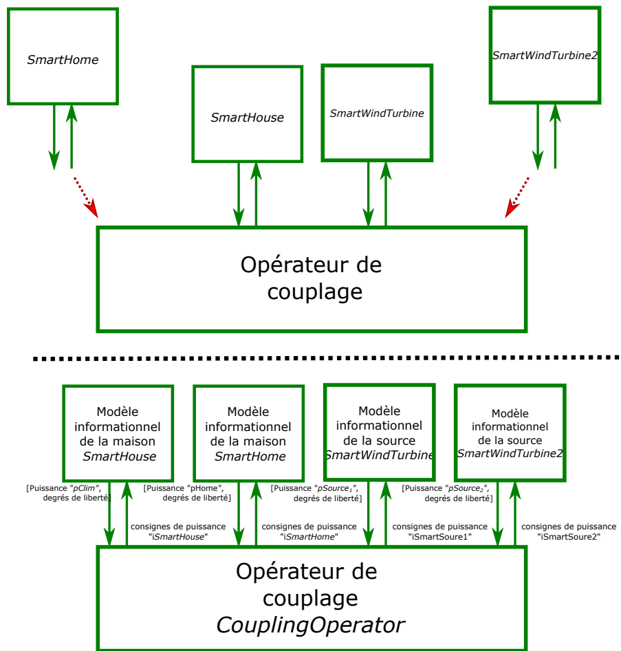
FIGURE 6.10 – Ajout de deux composants au multi-modèle 6.6.
