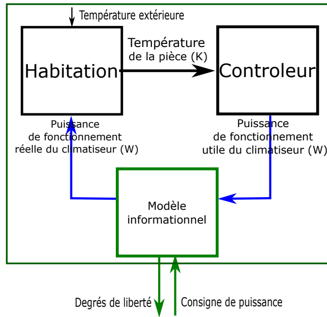
FIGURE 6.5 – Modèle thermique couplé informationnel.
