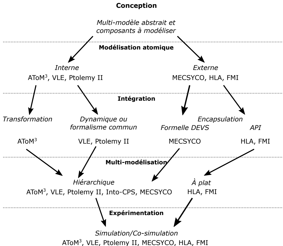
FIGURE 2.7 – Intergiciels placés selon leur approche de co-simulation utilisée, repris de [?]
