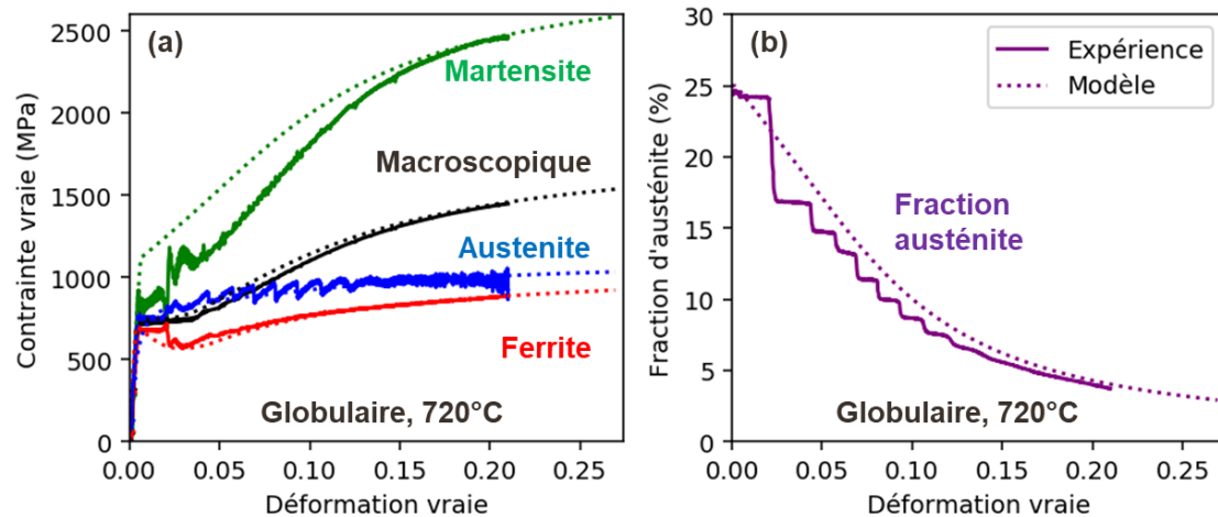
Figure 6: (a) Comparaison des contraintes d'écoulement mesurées expérimentalement (ligne continue) et calculées par le modèle (ligne en pointillé) dans la ferrite (rouge), l'austénite (bleu), la martensite (vert) et de la contrainte macroscopique (noir) de la microstructure globulaire recuite à 720°C. (b) Evolution de la fraction d'austénite dans la même expérience.
