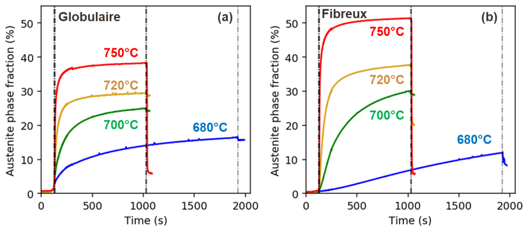
Figure 3: Evolution temporelle de la fraction de phase en austénite au cours des traitements thermiques pour les microstructures globulaires (a) et fibreuses (b). La température de recuit est indiquée sur chaque courbe. La première ligne verticale noire représente le début de la chauffe, la deuxième ligne correspond au début du refroidissement dans les aciers recuits au-dessus de 700°C (15 min) et la troisième ligne à celle du recuit à 680°C (30 min).
