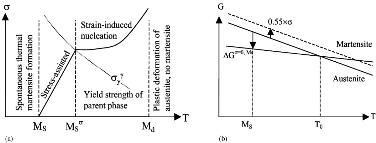
Figure 2 : (a) Evolution de la contrainte \sigma à appliquer à l'austénite pour déclencher la transformation martensitique, en fonction de la température. Les différents régimes de transformation sont indiqués. (b) Evolution schématique de l'énergie de Gibbs de l'austénite G^{\gamma} et de la martensite G^{\alpha'} en fonction de la température. L'effet d'une contrainte appliquée sur G^{\gamma} est indiqué en ligne pointillée [8].
