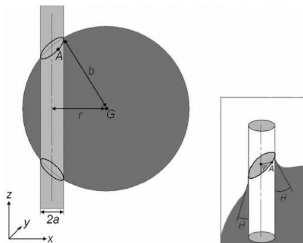
Figure 23 : Diagramme d'une gouttelette en forme de clam-shell (sphérique) sur une fibre, avec centre de masse (G) déplacé d'une distance r de la position axisymétrique. Le point A fait référence à un point arbitraire sur la ligne de contact, avec le paramètre \psi position de mesure sur le cercle de contact (voir encadré). Chaque point sur la ligne de contact posséderait un angle de contact gouttelette-fibre correspondant, ( \vartheta ), mesuré parallèle à l'axe des fibres [37].
