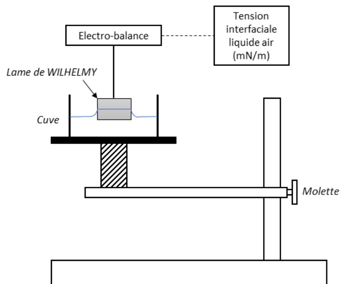
Figure 110 : Schéma du tensiomètre.
