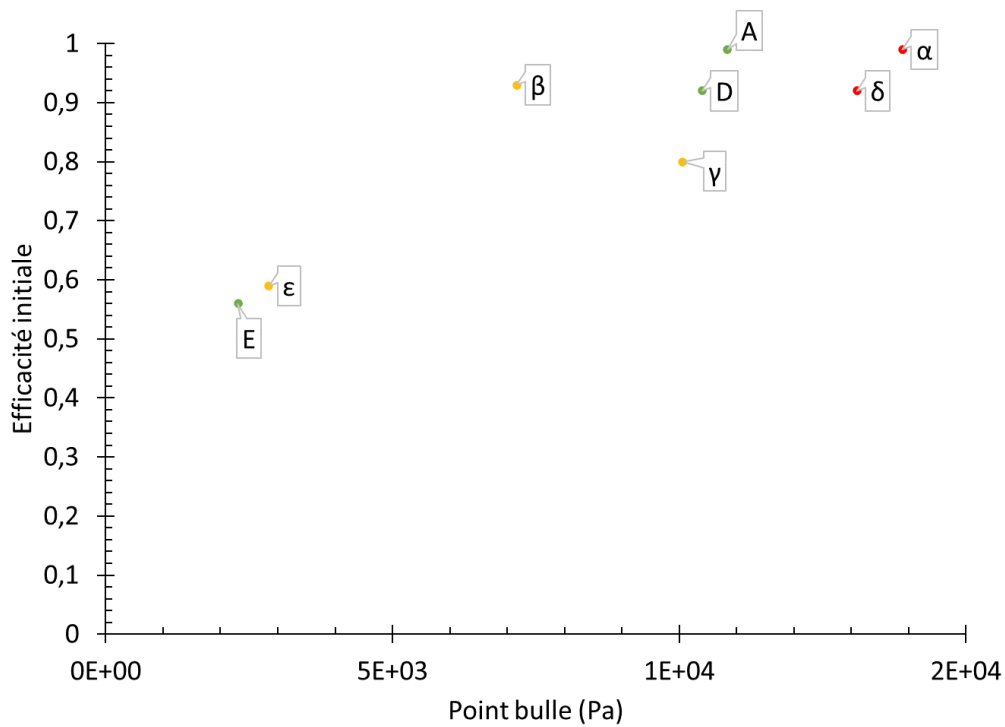
Figure 84 : Efficacité initiale en fonction du point bulle pour les différents filtres (en vert les filtres monocouches, en rouge les filtres multicouches symétriques et en jaune les filtres multicouches asymétriques).
