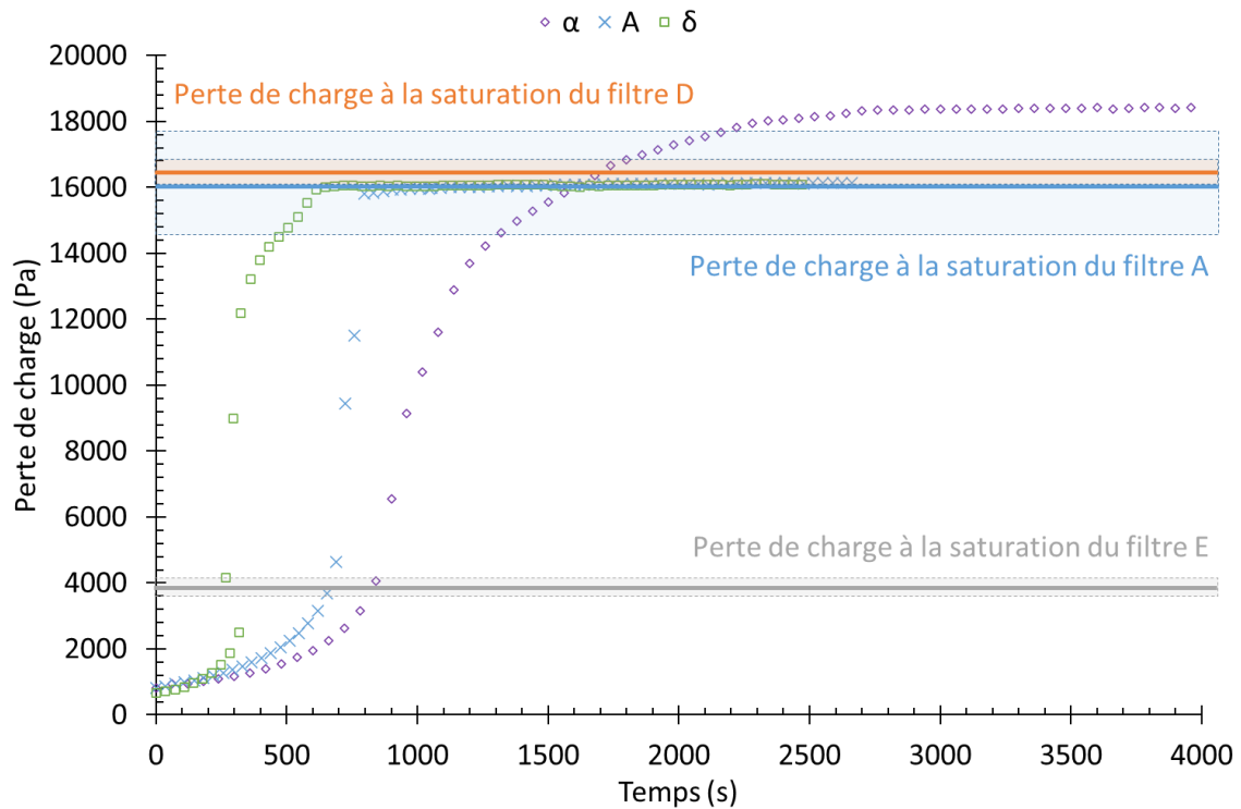
Figure 66 : Evolution de la perte de charge en fonction du temps, pour les filtres multicouches symétriques et le monocouche A, à une vitesse de filtration de 7 cm/s.
