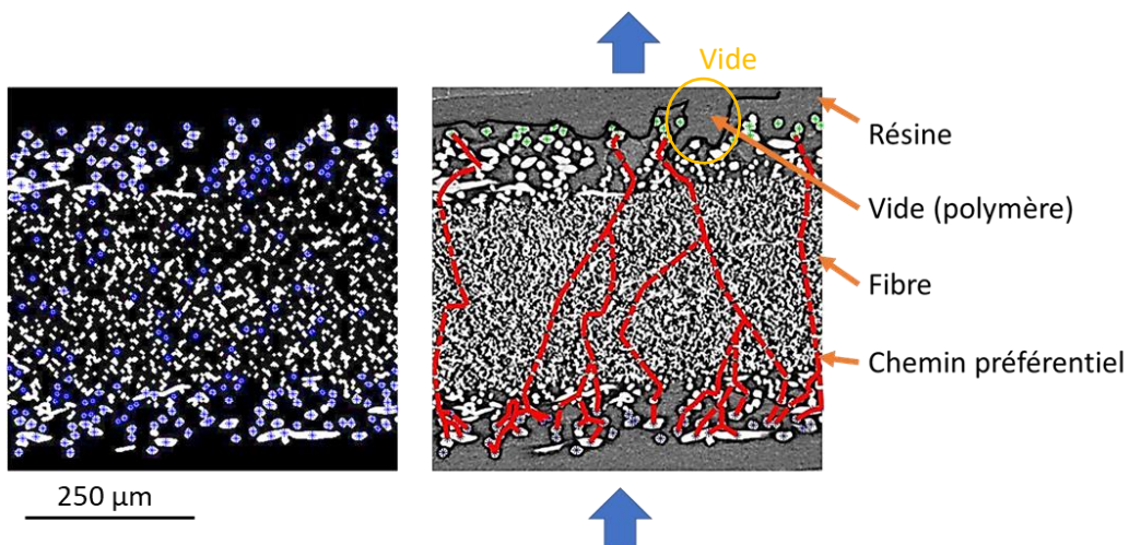
Figure 92 : Détection des chemins préférentiels du filtre \alpha , colmaté avec de la résine SU8_2002 (vitesse de filtration 7 cm/s) (l'image de gauche correspond aux fibres qui sont détectées, en bleu, et l'image de droite correspond aux chemins préférentiels qui sont calculés, en rouge).
