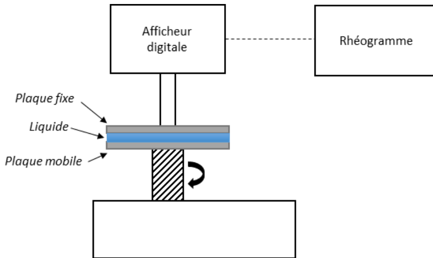
Figure 101 : Schéma de mesure de la viscosité
