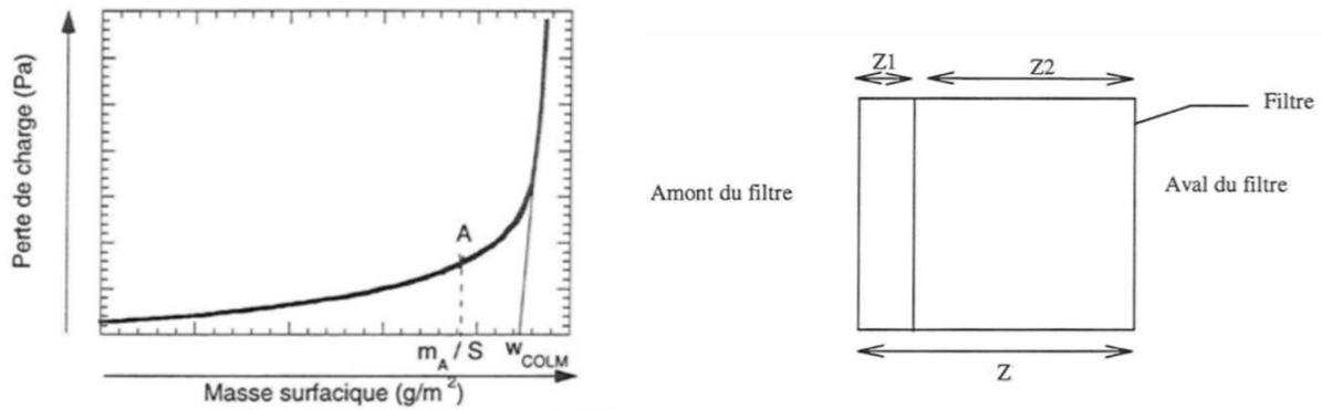
Figure 32 : Evolution de la perte de charge en fonction de la masse surfacique, avec le point A de transition (à gauche), et schématisation de la décomposition du filtre [42].
