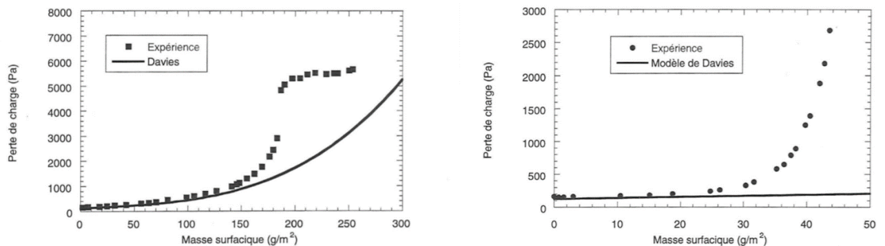
Figure 31 : Comparaison du modèle de Davies avec les points expérimentaux décrivant l'évolution de la perte de charge en fonction de la masse surfacique, pour un aérosol mouillable (aérosol DMP, à gauche), et un non-mouillable (aérosol de glycérol, à droite) [42].
