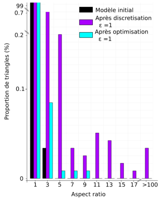
FIGURE 2.15 – Distribution de la qualité des triangles au cours des étapes d'édition du maillage avec l'optimisation des intersections.
