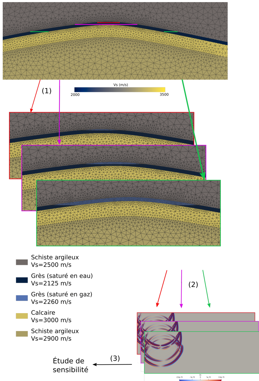
FIGURE 3.1 – Modifications du maillage d’une couche géologique pour la détermination de la profondeur d’un contact fluide à partir de données sismiques. (1) À partir de plusieurs isovaleurs du champ scalaire, les positions possibles du contact gaz-eau sont maillées grâce à notre méthode de remaillage local. (2) Le logiciel Hou10ni2D [Barucq, 2016] est ensuite utilisé pour simuler la propagation des ondes afin (3) d’étudier la sensibilité des données sismiques à la profondeur du contact.
