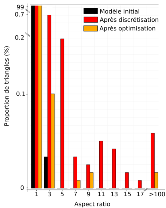
FIGURE 2.12 – Distribution de la qualité des triangles lors de l'insertion d'une ligne. Cette mesure est calculée sur les modèles Figure 2.11a. et b.
